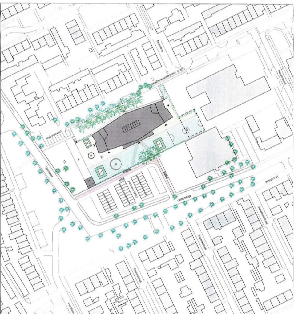
Situatie Nieuw
