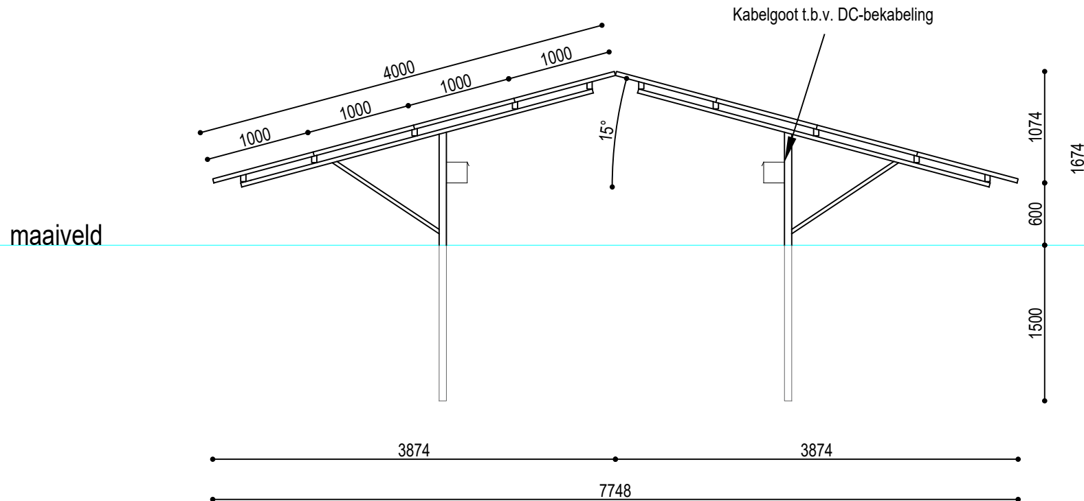
Detail constructie 1:50
