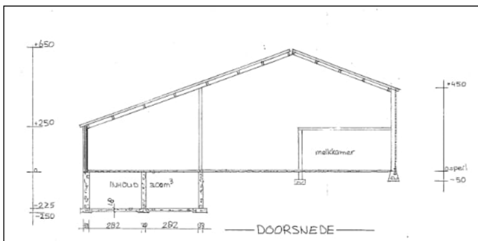
Figuur 20: Uitsnede bouwtekening bedrijfsgebouw met mestkelder
