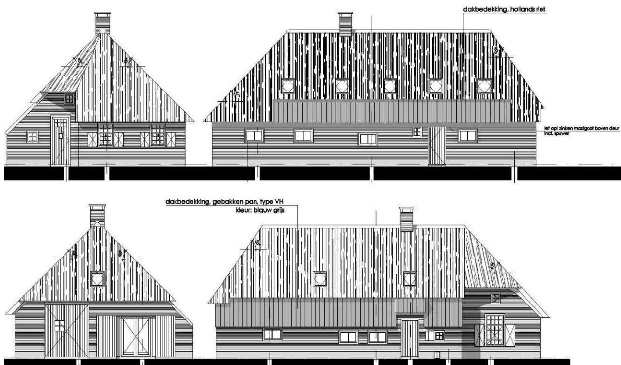
Afbeelding 3.3. Schets nieuw te bouwen woonhuis (IN Bouwkunde en vormgeving, 2011).
