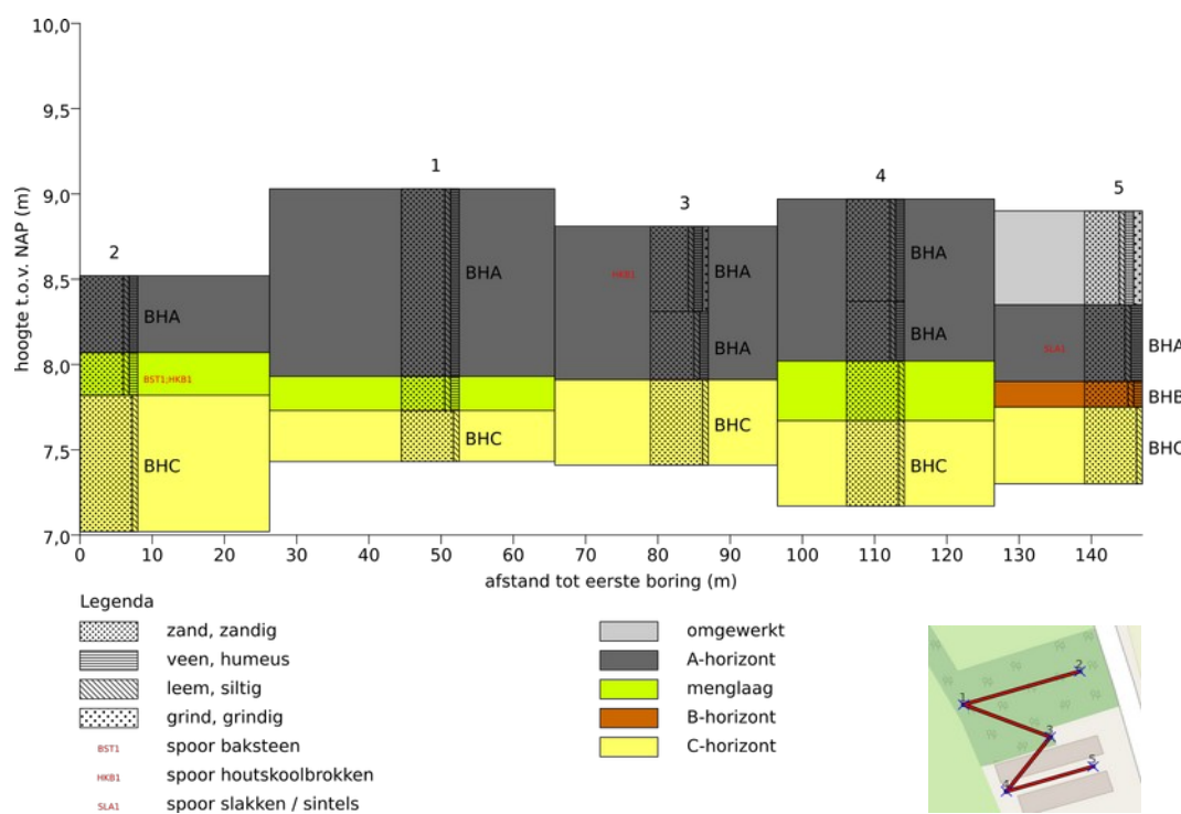
Figuur 26: Getekende boorprofielen in schematische doorsnede, en aanduiding van bodemhorizonten.
