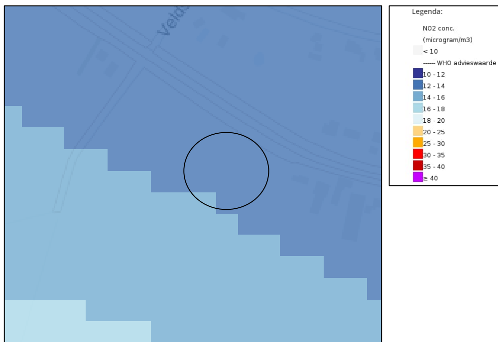
Figuur 24: Stikstofoxide 2020 NO 2 (bron: Atlas leefomgeving, RIVM) waarop de ligging van het plangebied is aangeduid
