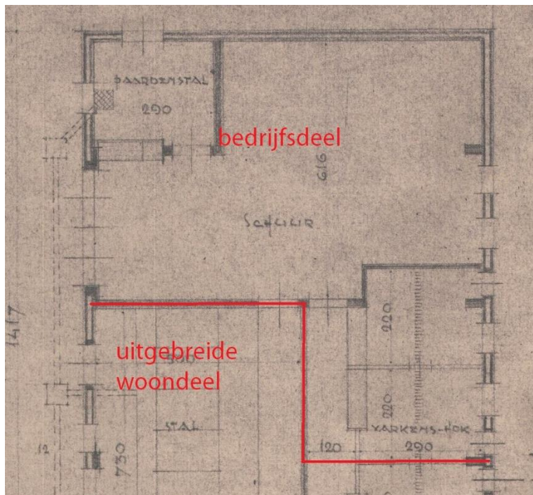
Plattegrond bouwtekening 1951. De rode lijn geeft de nieuwe scheiding tussen woon- en bedrijfsdeel aan
