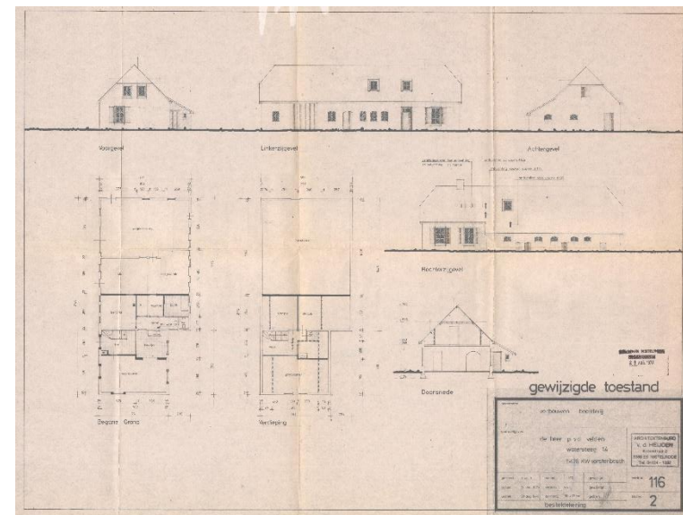
Bouwtekening verbouw boerderij in 1978. Bron: BHIC
