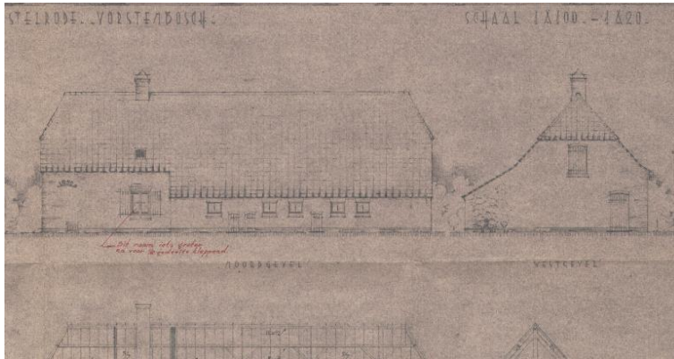
Gevels bouwtekening 1951
