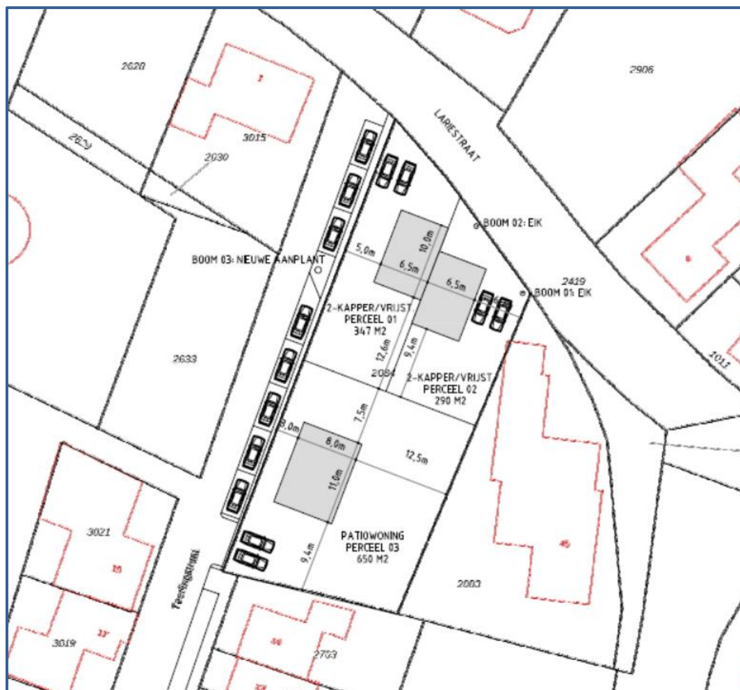
Afbeelding 2. Situatietekening beoogde situatie
