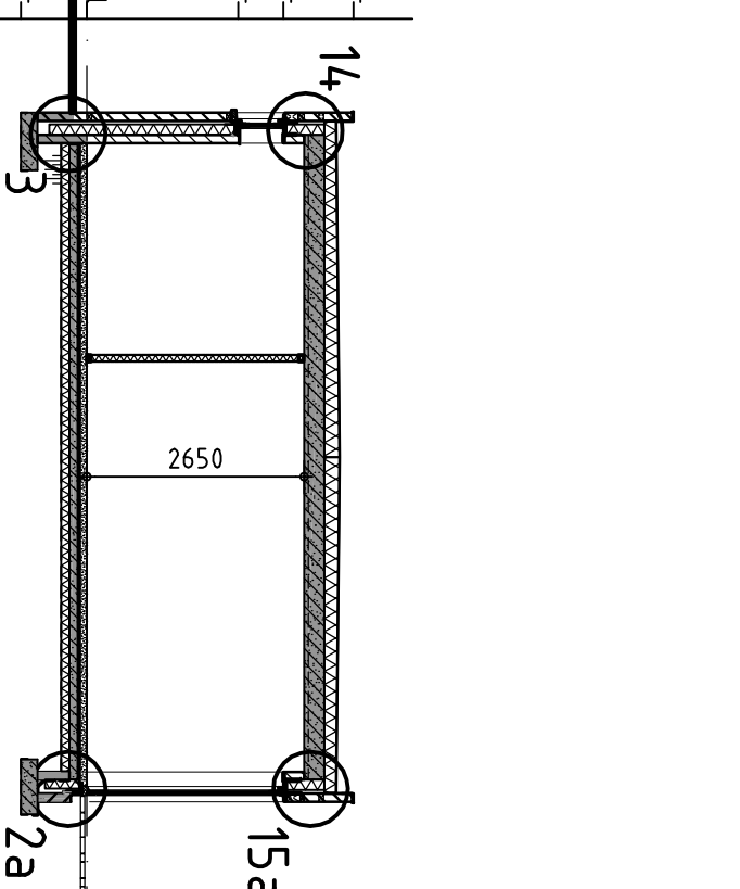
Doorsnede B-B
