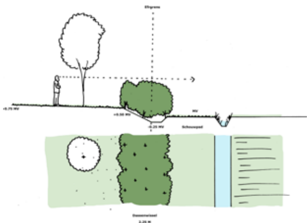
Doorsnede dassenwissel/kavelgrens
