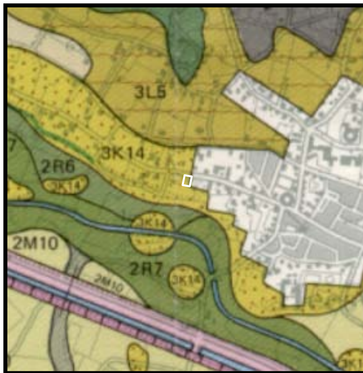
Figuur 3: Een deel van de geomorfologische kaart waarop het plangebied wit omkaderd is. Het plangebied ligt binnen een zone die met kaartcode 3K14 is aangegeven, wat betekent dat het plangebied is gelegen op een dekzandrug met al dan niet een oud bouwlanddek.
