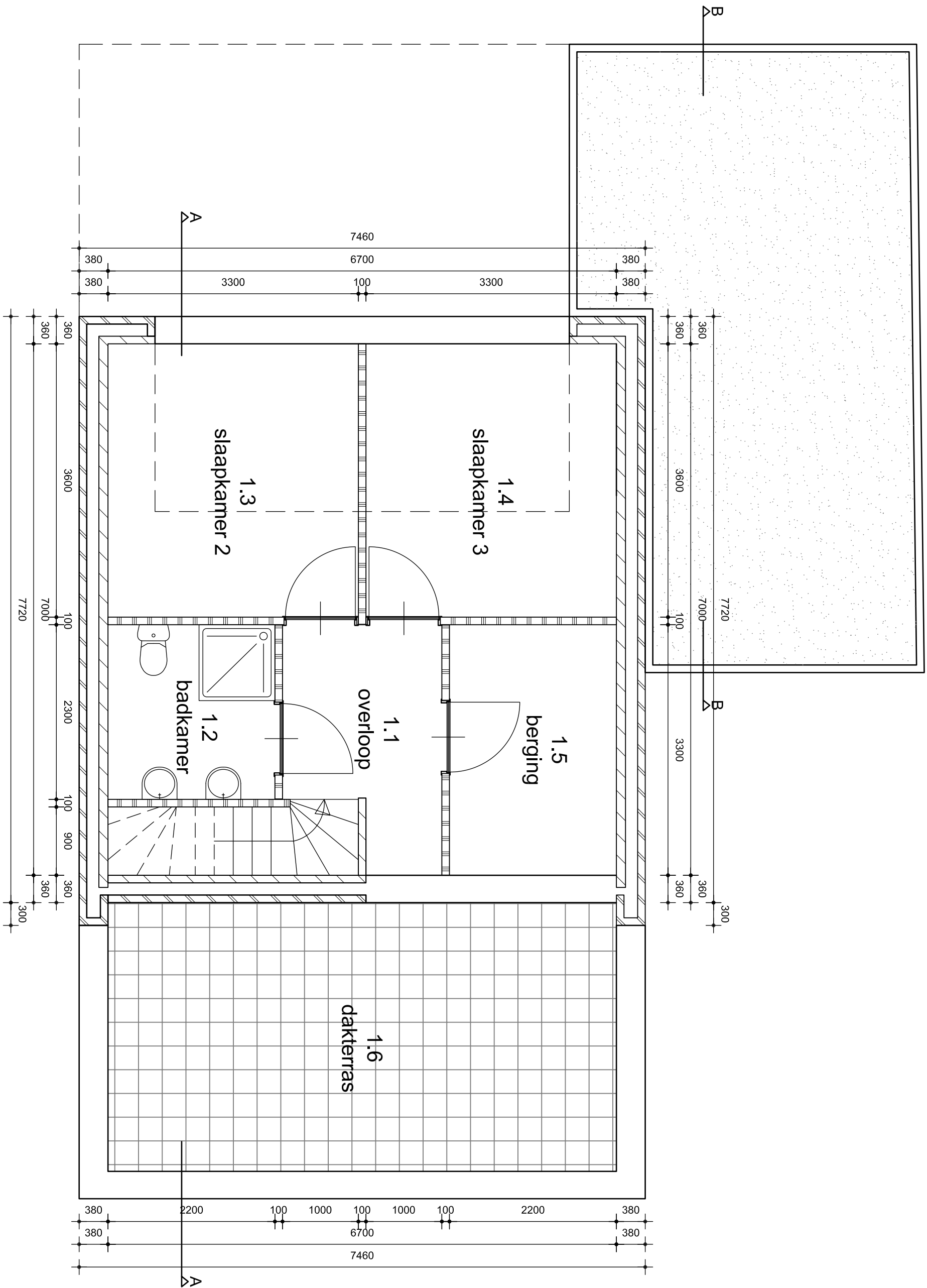
Plattegrond verdieping
