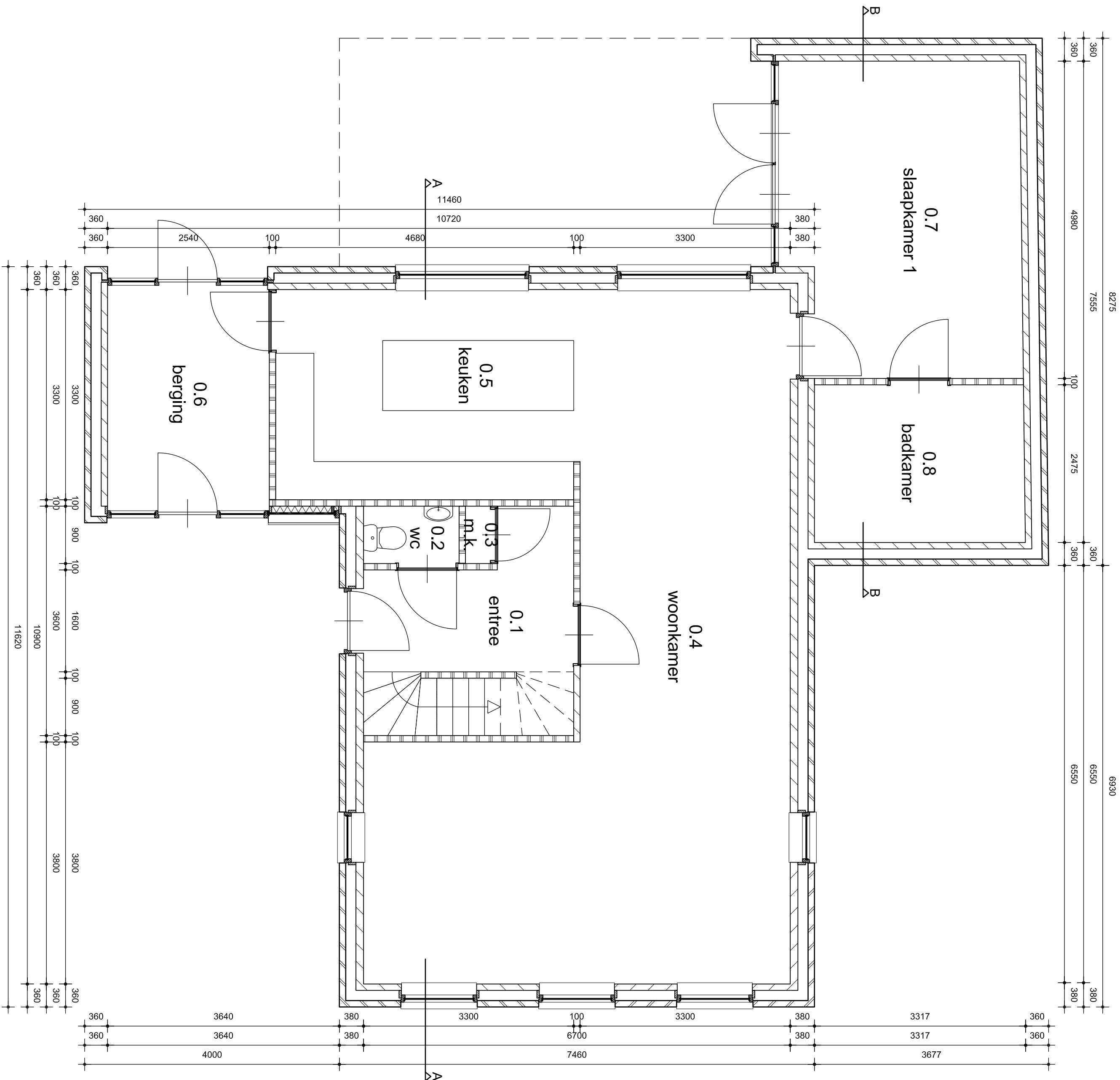
Plattegrond begane grond
