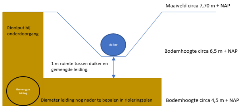
Afbeelding 27 Schetsmatige weergave kruising gemengde leiding met waterloop
