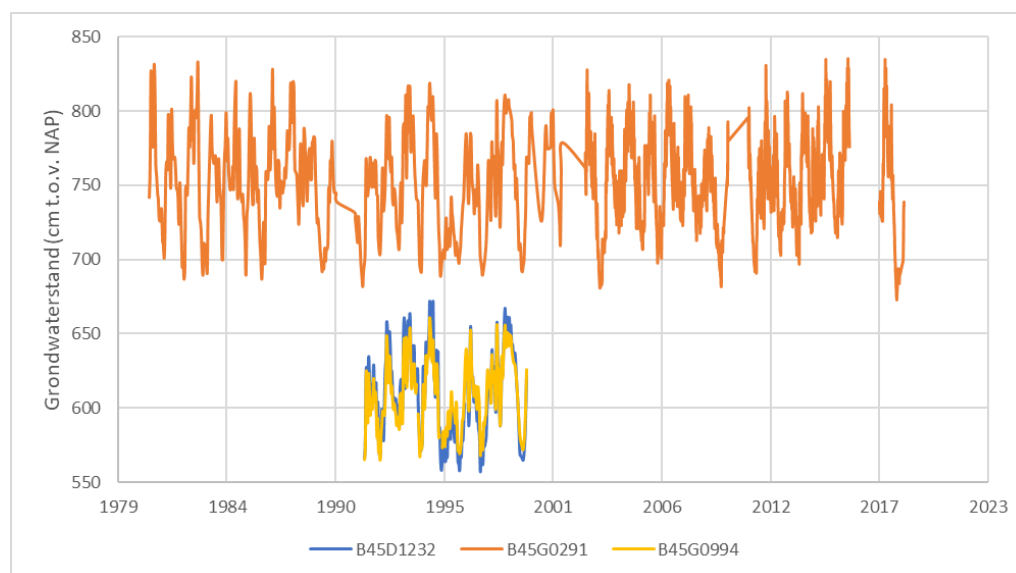
Afbeelding 8 Grondwaterstanden van peilbuizen in de omgeving van het plangebied
