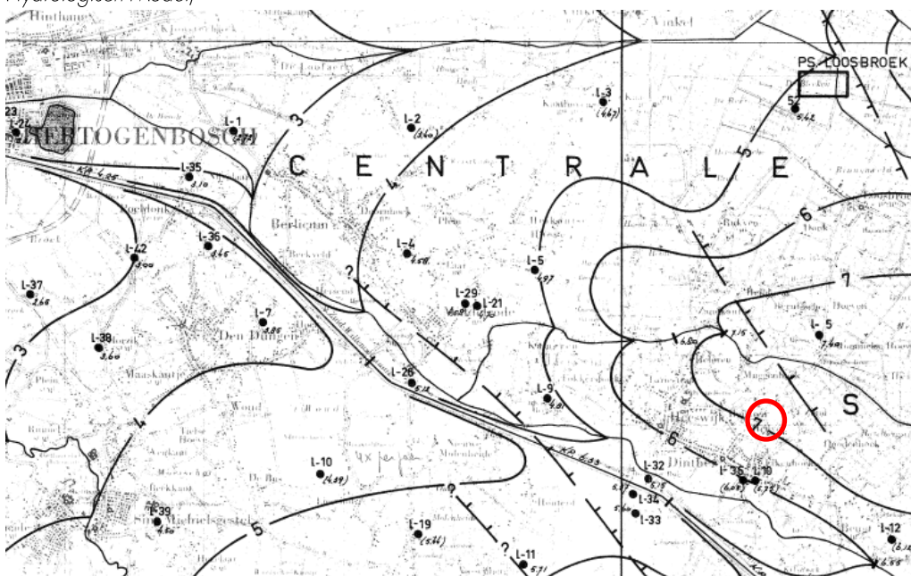
Afbeelding 6 Grondwaterkaart van Nederland met in de rode cirkel de globale locatie van het plangebied
