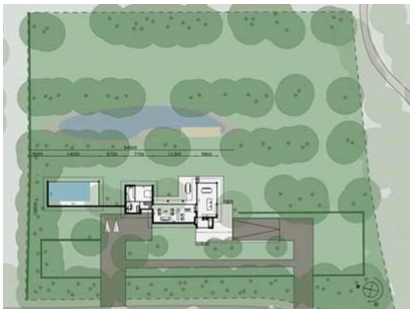
Figuur 3.1. Tekening van de toekomstige situatie. Bron: CroonenBuro5.
