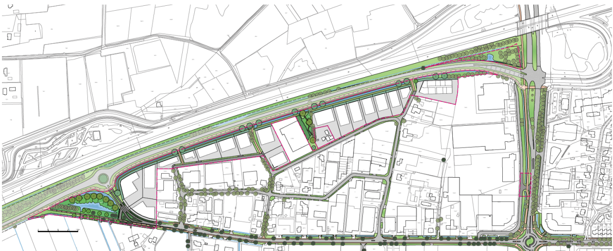
Figuur 6.2 Ontwerp uit stedenbouwkundig plan volgens Cereslaan-West (Bron: Kuiper Compagnons/KruitKok Architecten)
