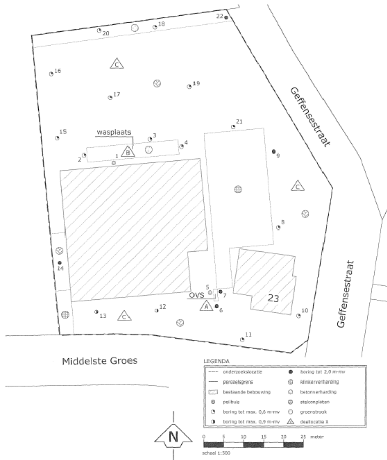
Afbeelding 2.4: Situatietekening locatie Middelste Groes 23 met ligging wasplaats (bron: Nulsituatie onderzoek, rapportnummer 20101122, d.d. 26-05-2010 door Milon)
