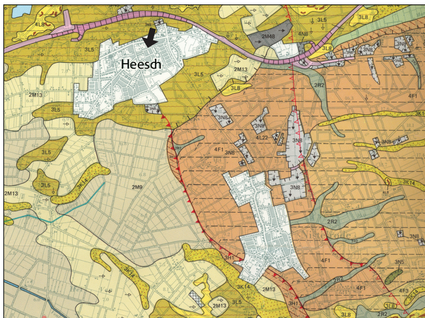
Figuur 2.1 Geomorfologische kaart van Heesch en omgeving met (in het rood) de breuklijnen
