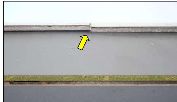
Figuur 14. Ruimte tussen daktrim en boeidelen van het bedrijfsgebouw.
