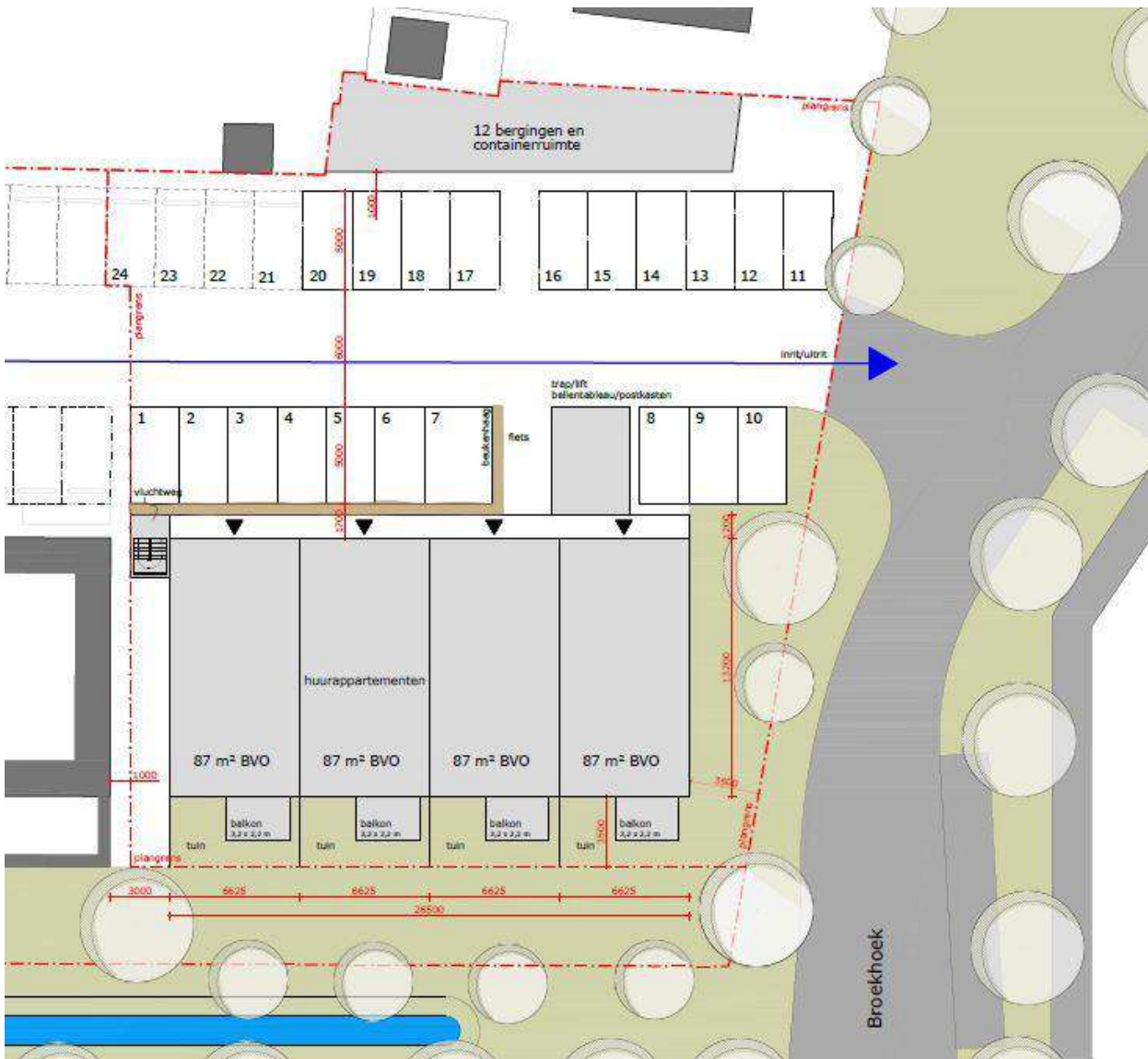
Figuur 2.5 Voorstel situering nieuwbouw en omgeving
