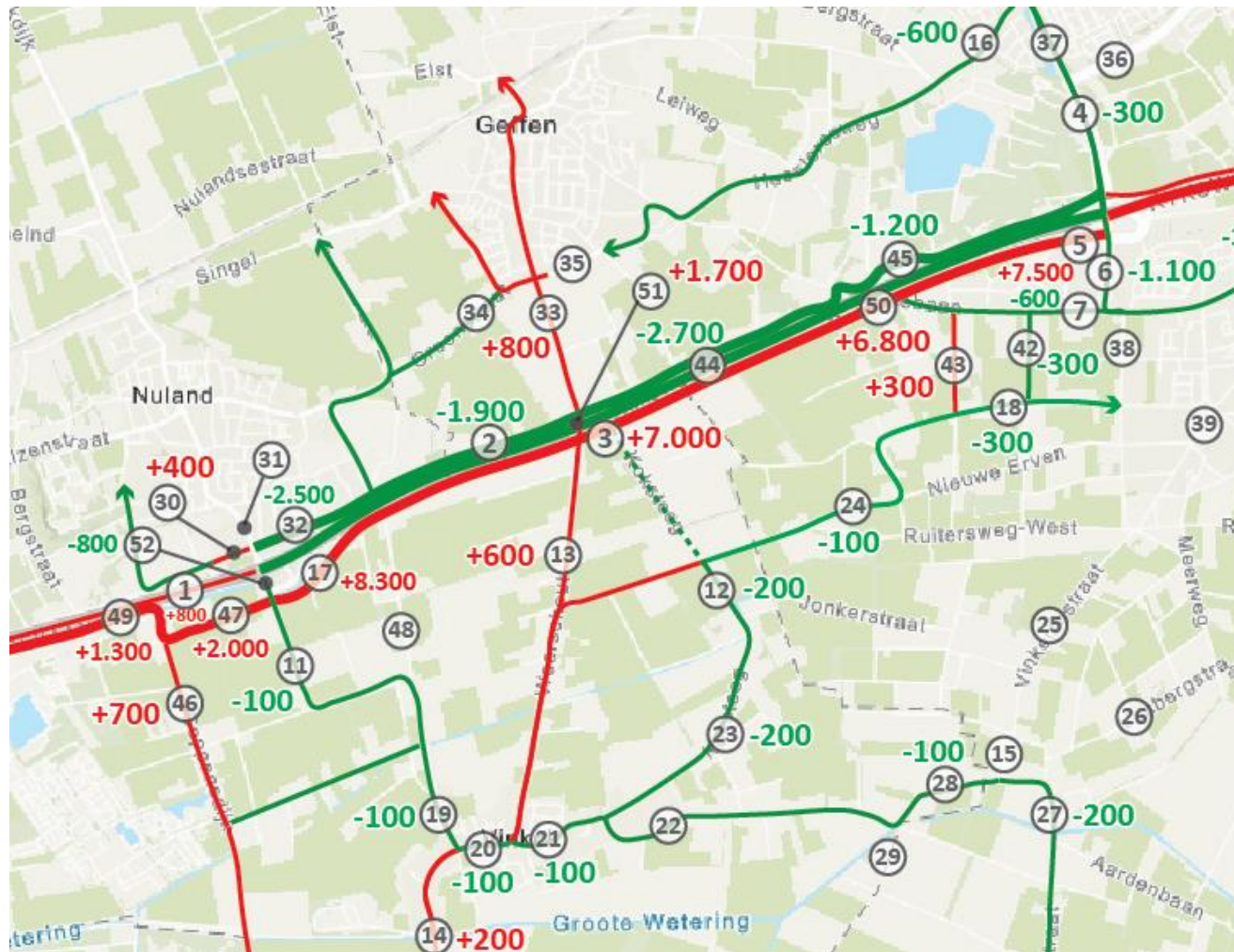
Toe- (rood) en afnames (groen) van verkeer (in mvt/etm) op de wegen rond Heesch West)
