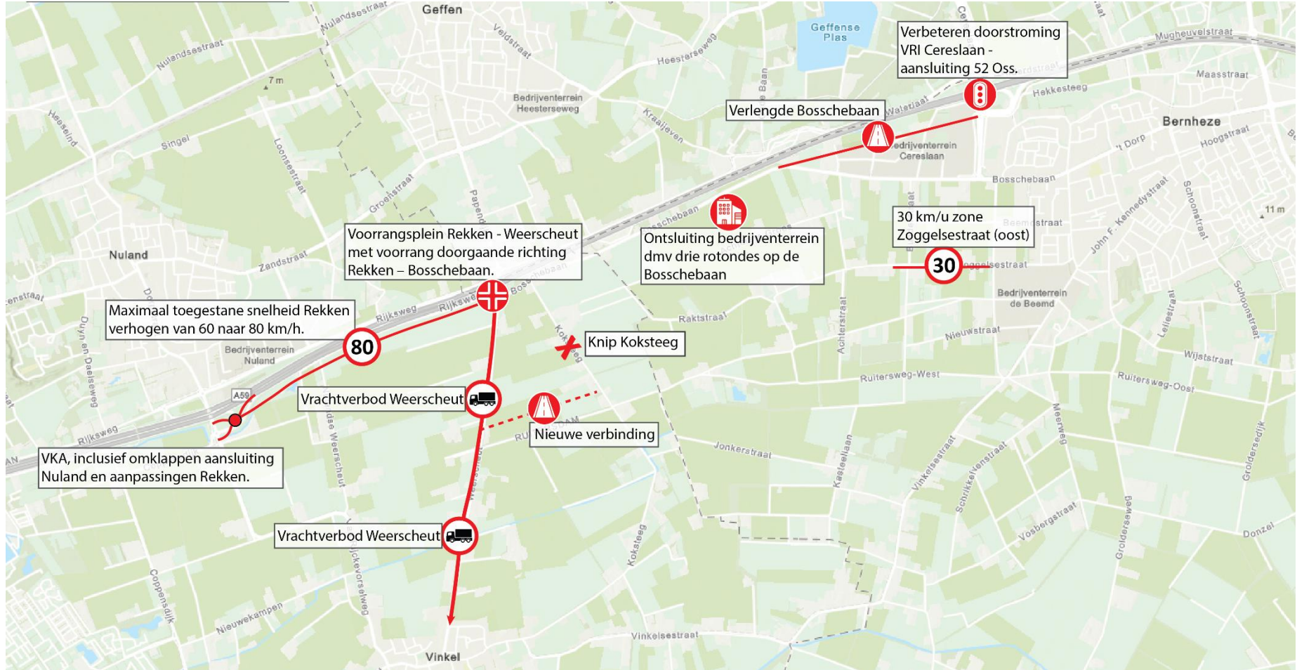
Totaaloverzicht verkeerskundige maatregelen Heesch West (maatregelen 2019 + aanvullende maatregelen 2021) (bron: Goudappel,2021)
