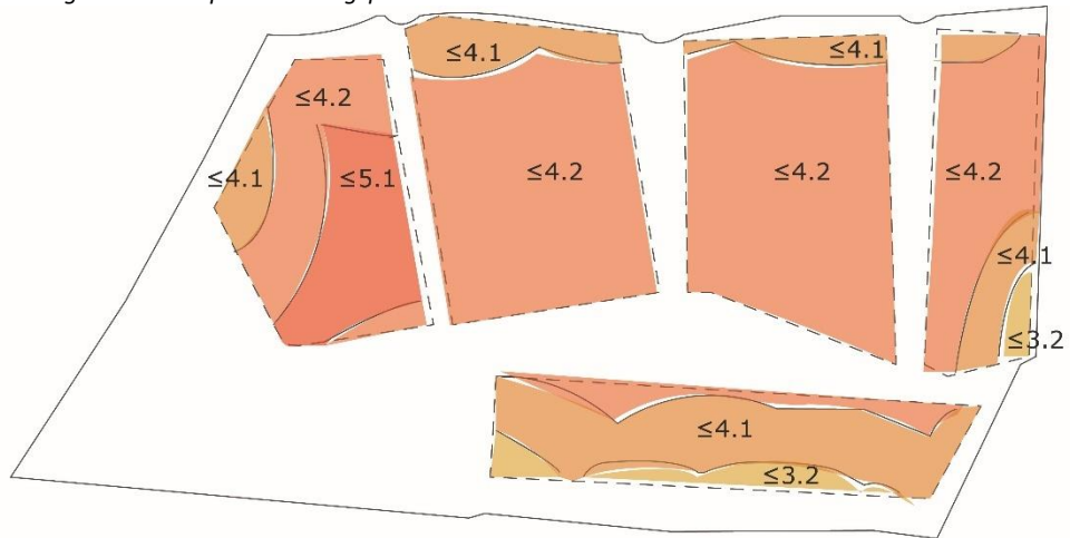
Milieuzonering ontwerpbestemmingsplan
