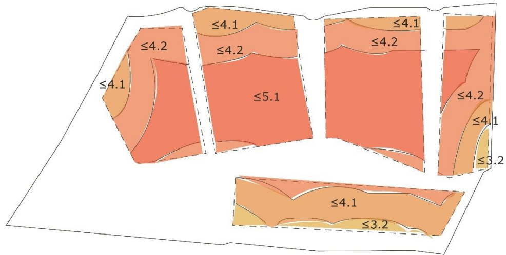
Milieuzonering voorontwerpbestemmingsplan
