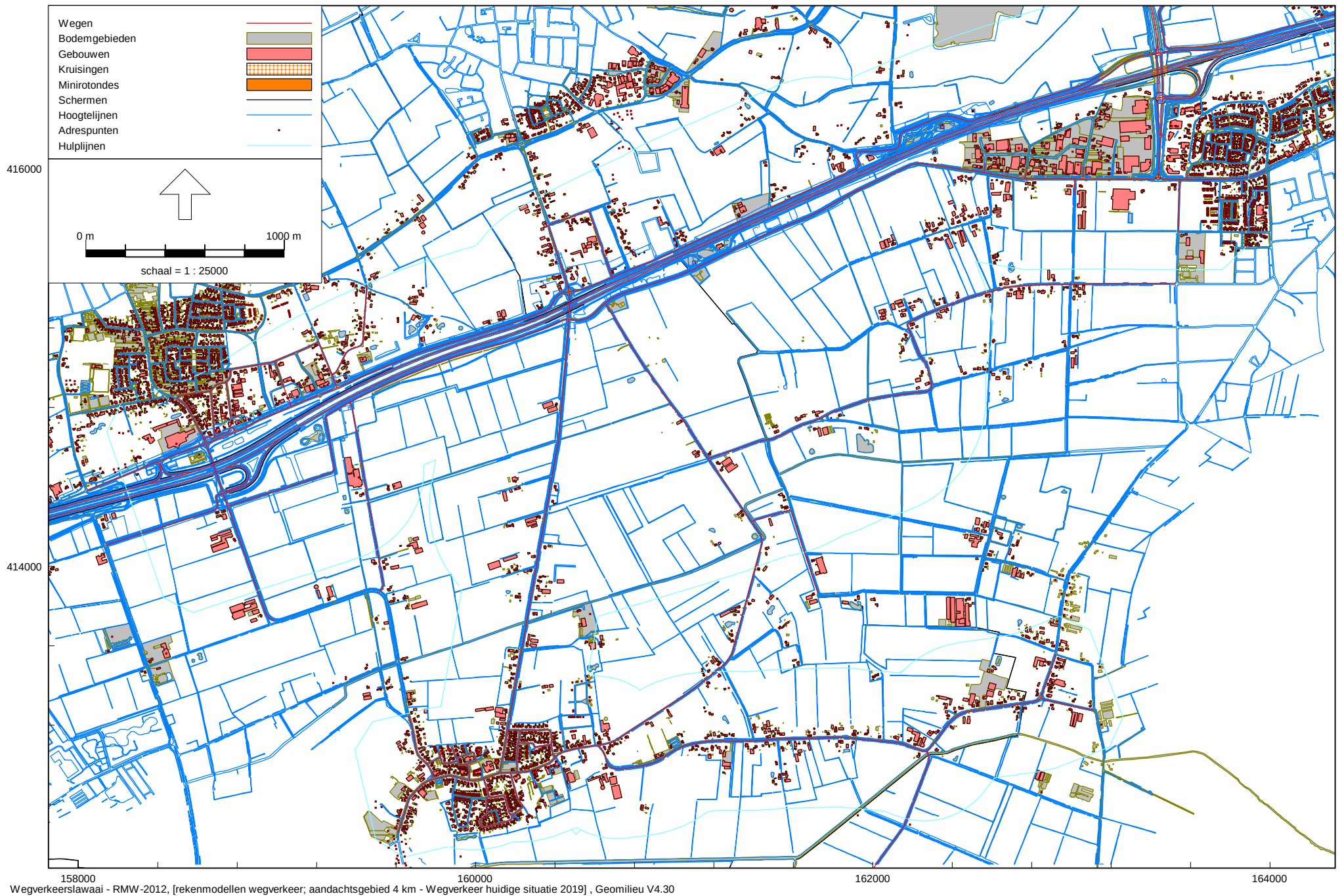
Overzicht rekenmodel wegverkeerslawai Heesch West Huidige situatie
