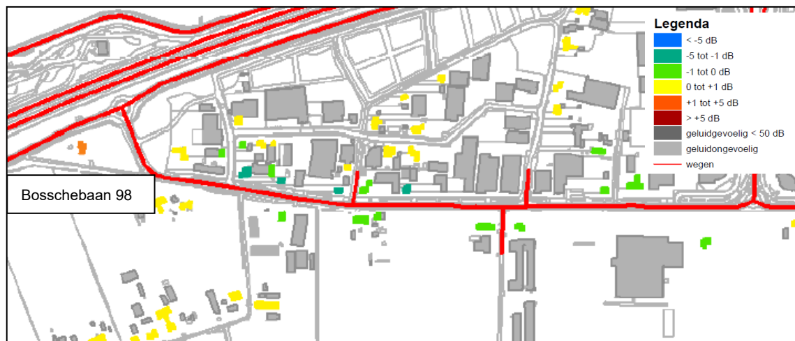
Afbeelding 4.11 : Akoestisch effect verlegging Bosschebaan (VKA versus autonoom).
