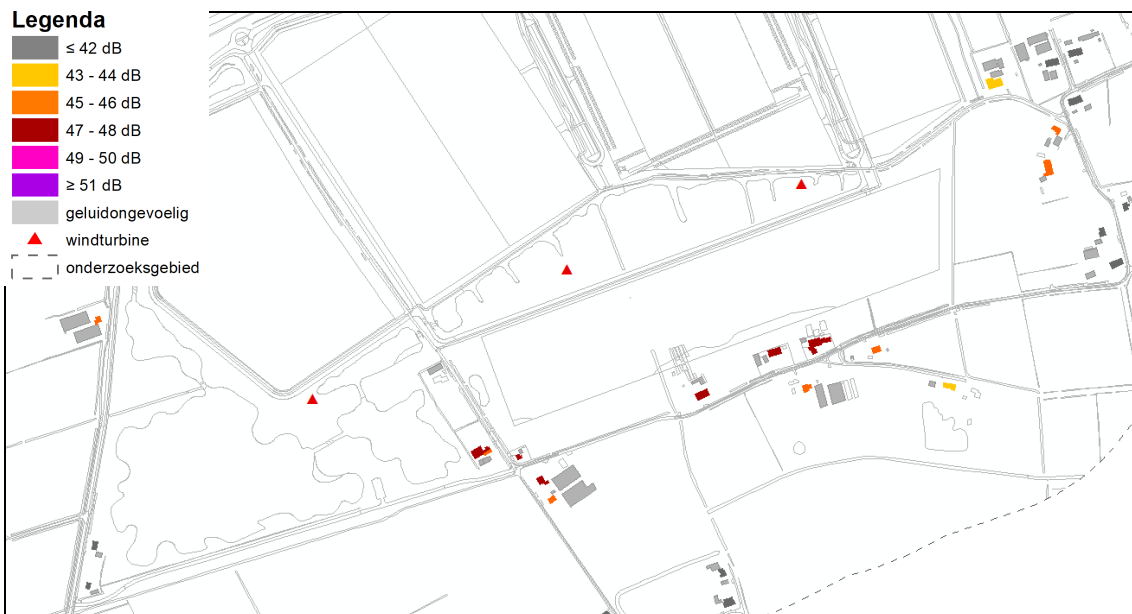
Afbeelding 4.14 : Akoestisch effect windturbinegeluid variant 1b met terugschakeling
