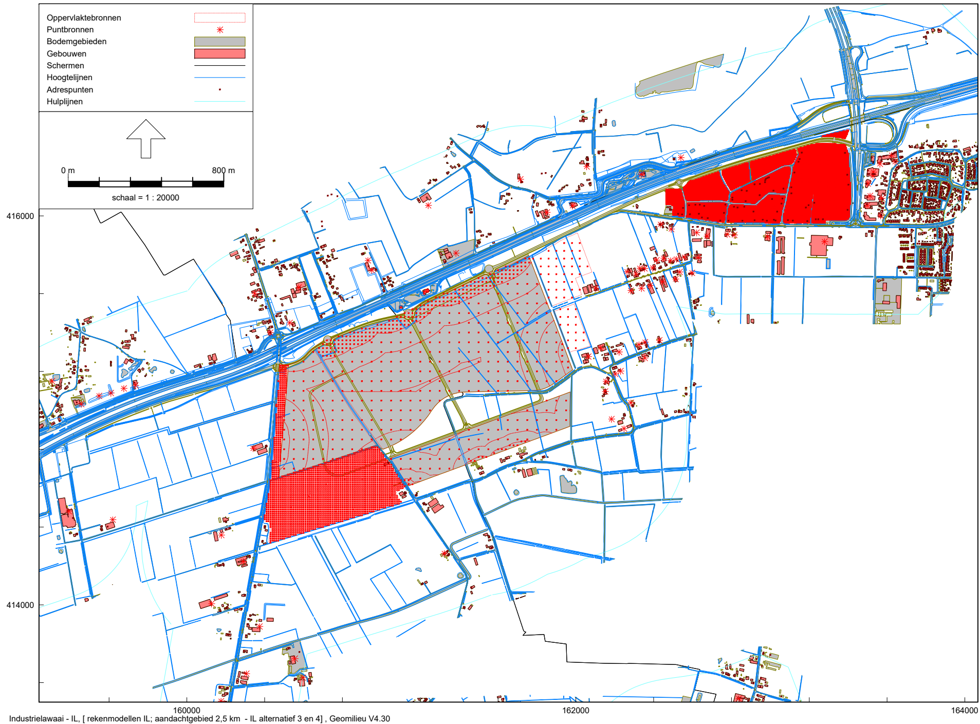
Overzicht rekenmodel industrielawaai Heesch West Alternatief 3 en 4
