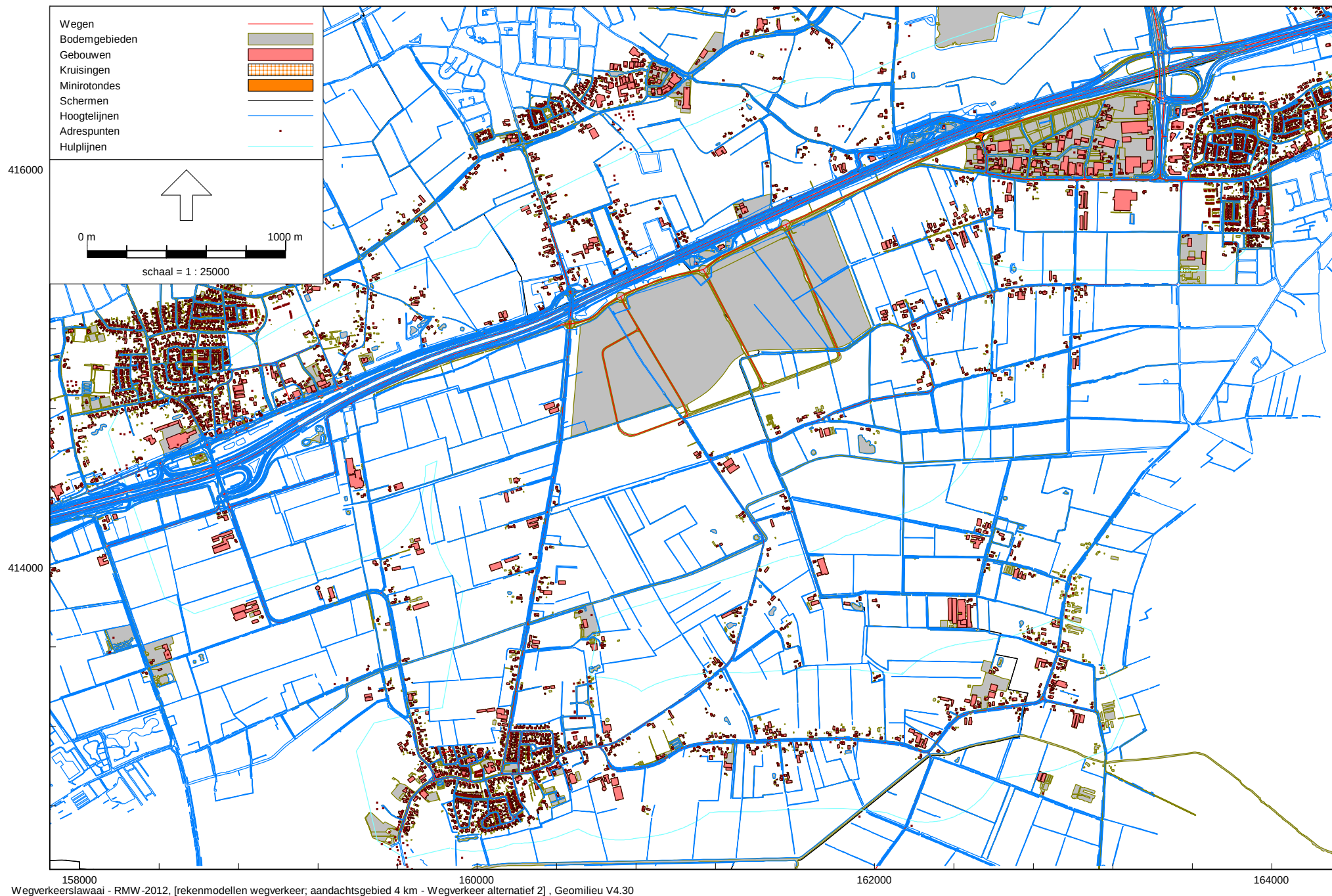
Overzicht rekenmodel wegverkeerslawaaï Heesch West Alternatief 1 en 2
