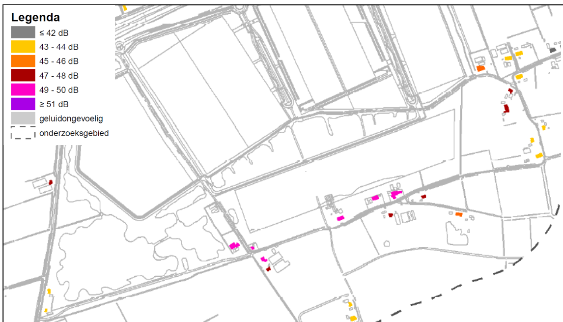
Afbeelding 4.8 : Akoestisch effect windturbinegeluid variant 1b
