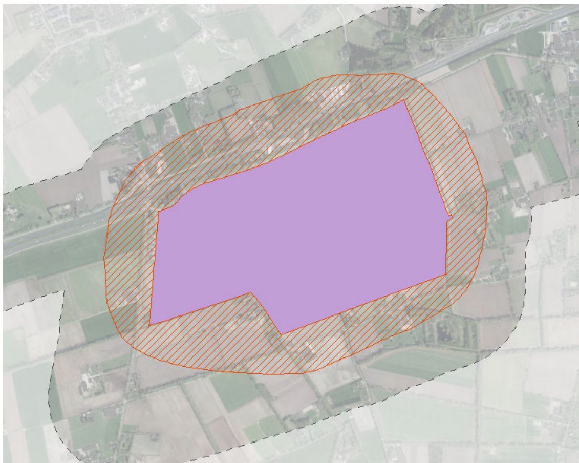
Afbeelding 4.5 : 50 dB contour (oranje arcering) industrieterrein Heesch-West alternatief 3 en 4.
