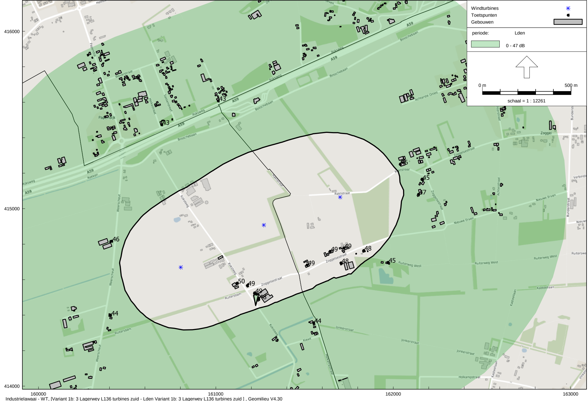
Lden VKA - Variant 1b: 3 Lagerwey L136 windturbines, ashoogte 132 meter, zuiden bedrijventerrein
