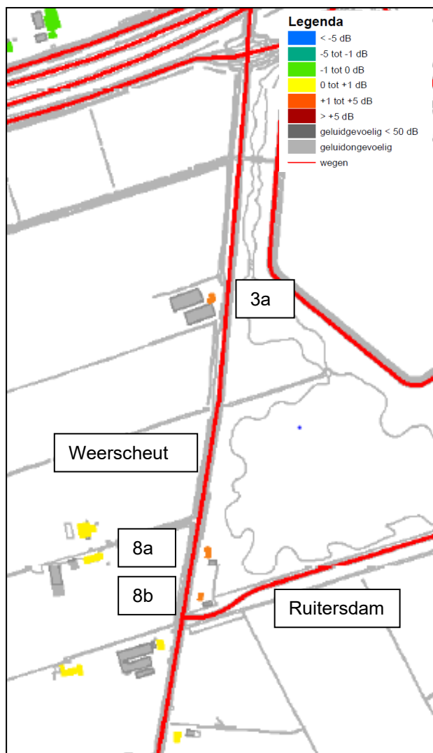
Afbeelding 4.12: Akoestisch effect Weerscheut (VKA versus autonoom)
