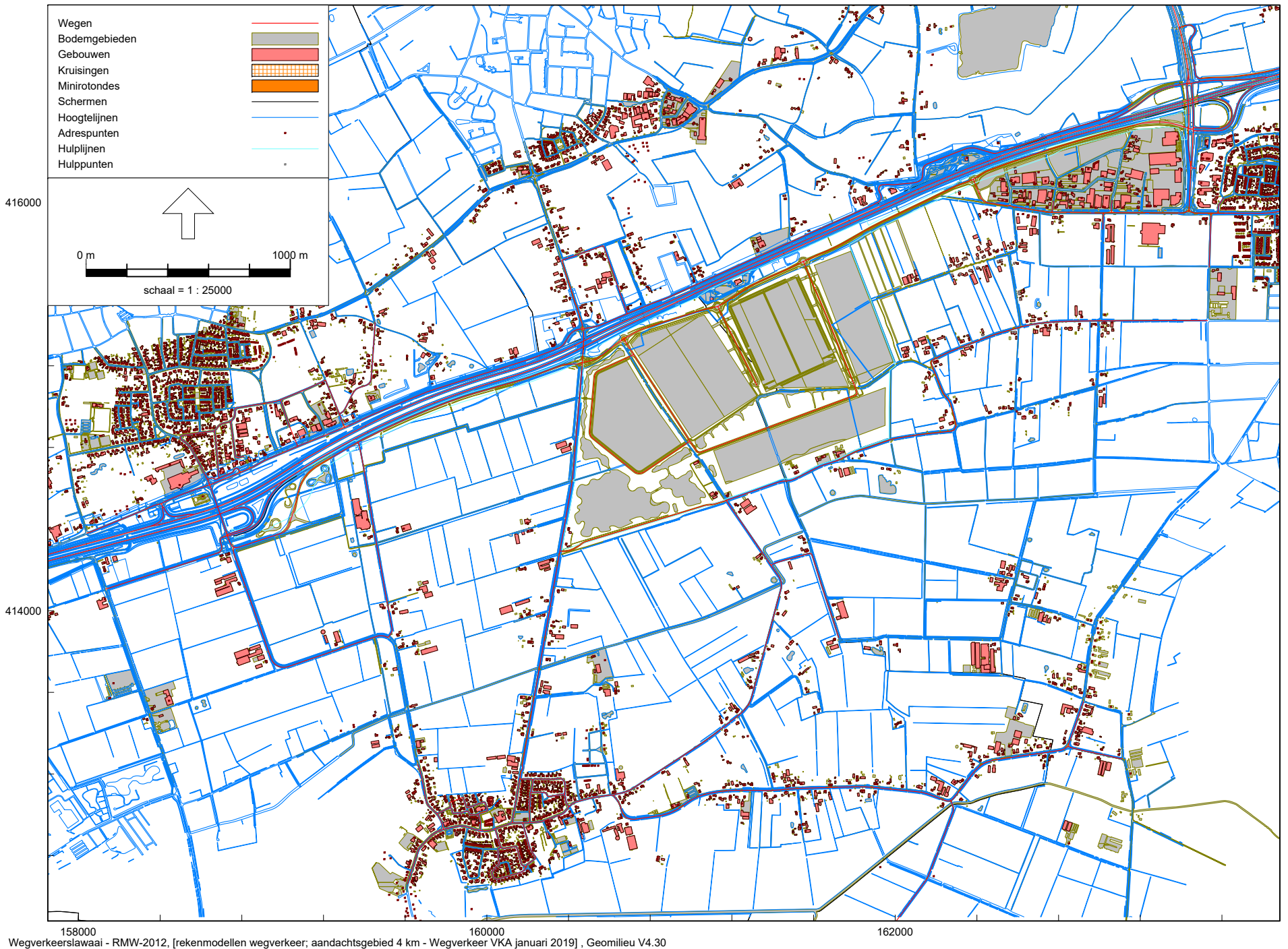
Overzicht rekenmodel wegverkeerslawaii Heesch West Voorkeursalternatief
