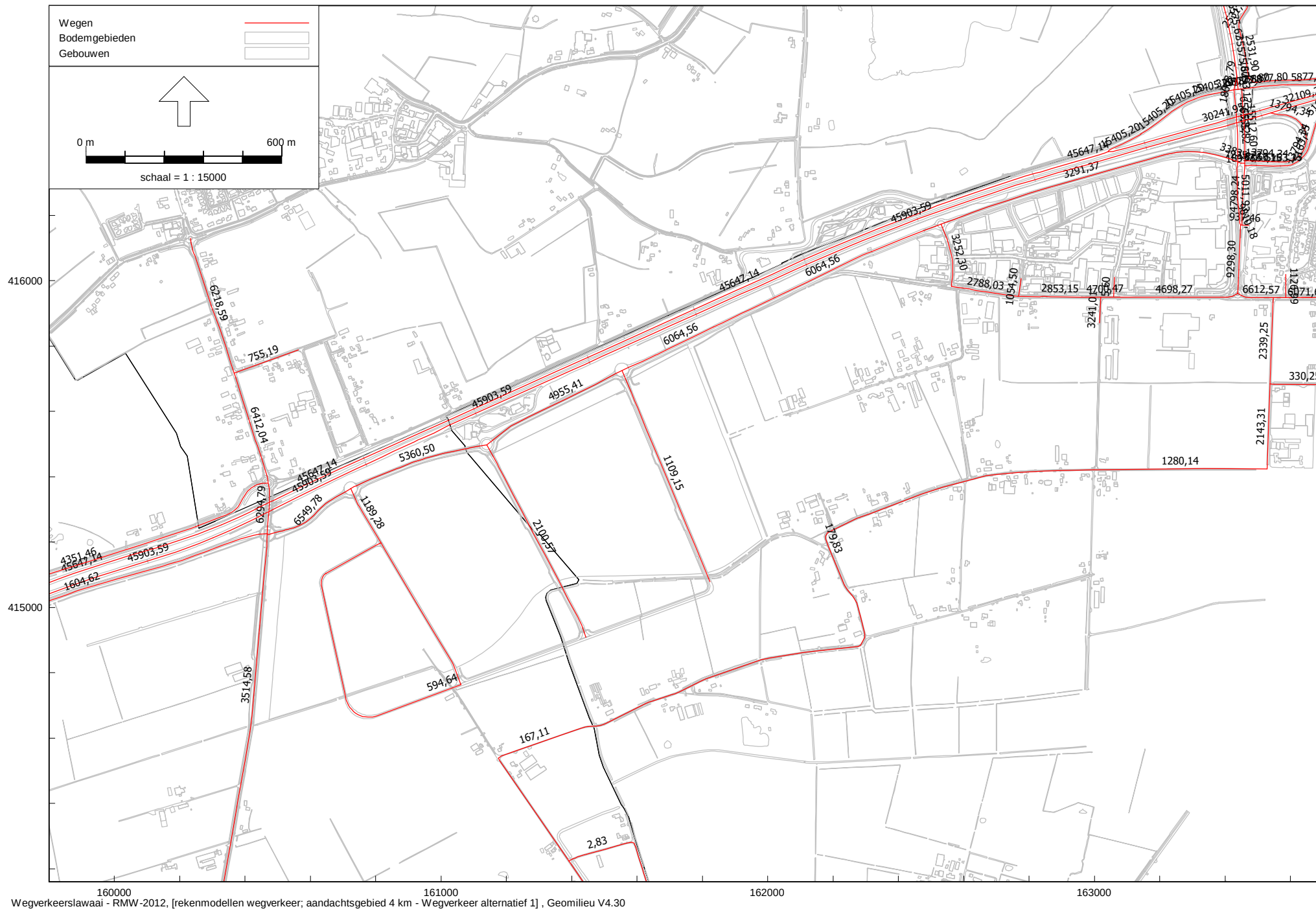
Verkeersintensiteiten alternatief 1
