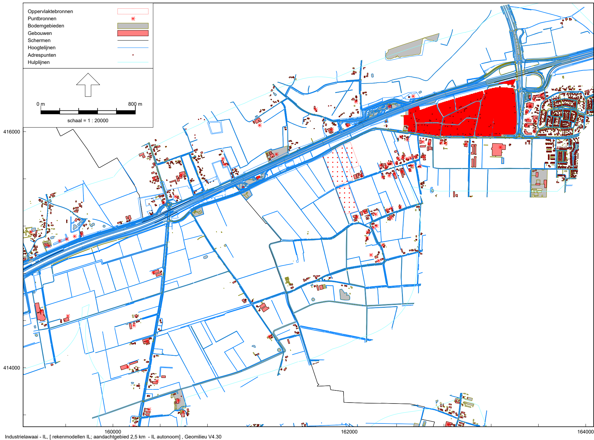
Overzicht rekenmodel industrielawaai Heesch West Autonoom
