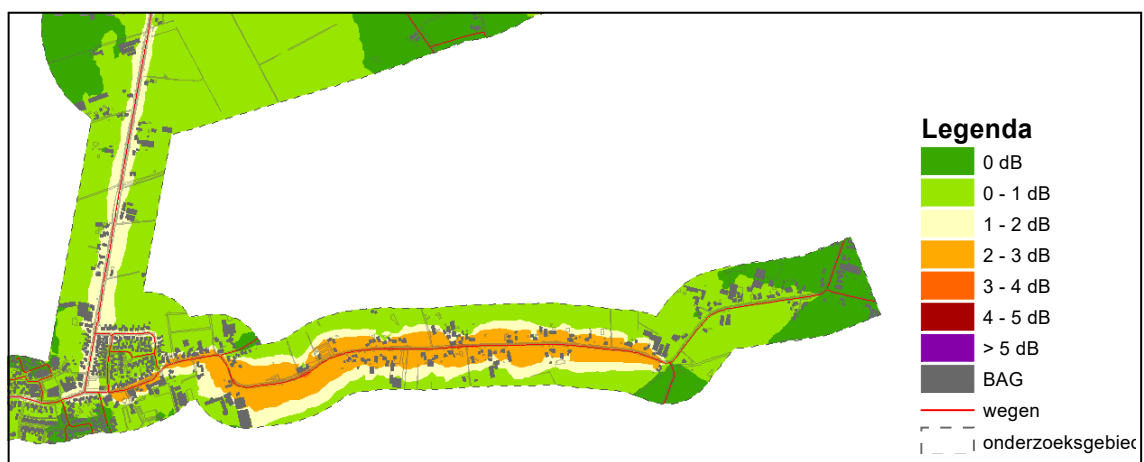
Afbeelding 4.3 : Weggedeelte Weerscheut, Lindenlaan en Vinkelseweg met toename geluidsbelasting (situatie alternatief 3 in vergelijking met autonoom)
