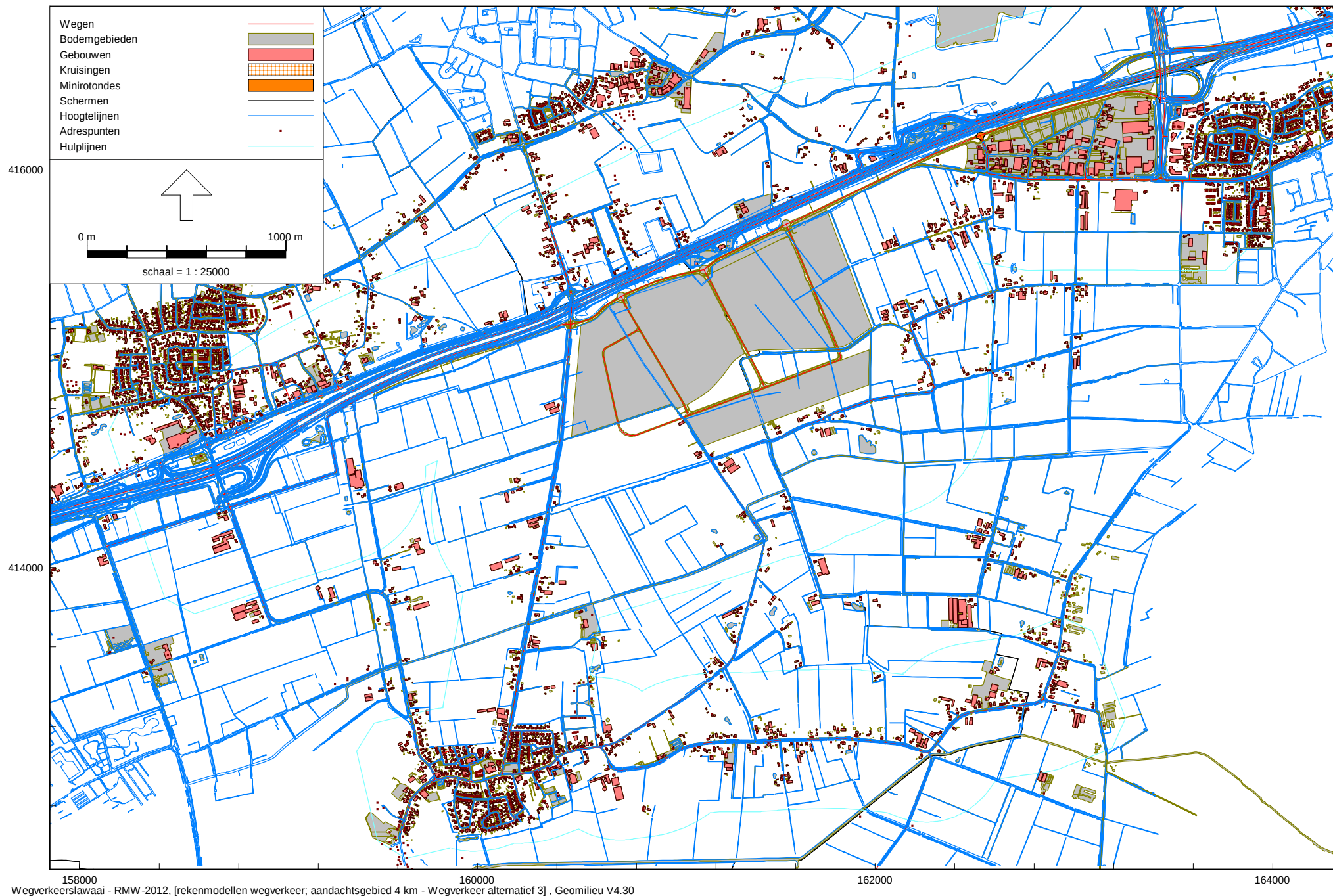
Overzicht rekenmodel wegverkeerslawai Heesch West Alternatief 3 en 4
