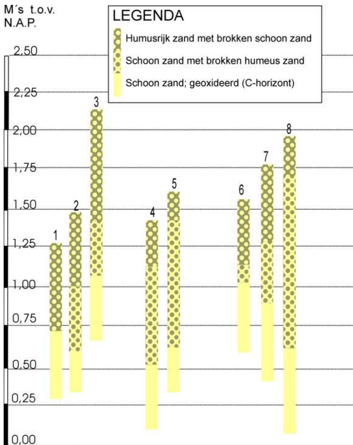
Figuur 19: Boorprofielen
