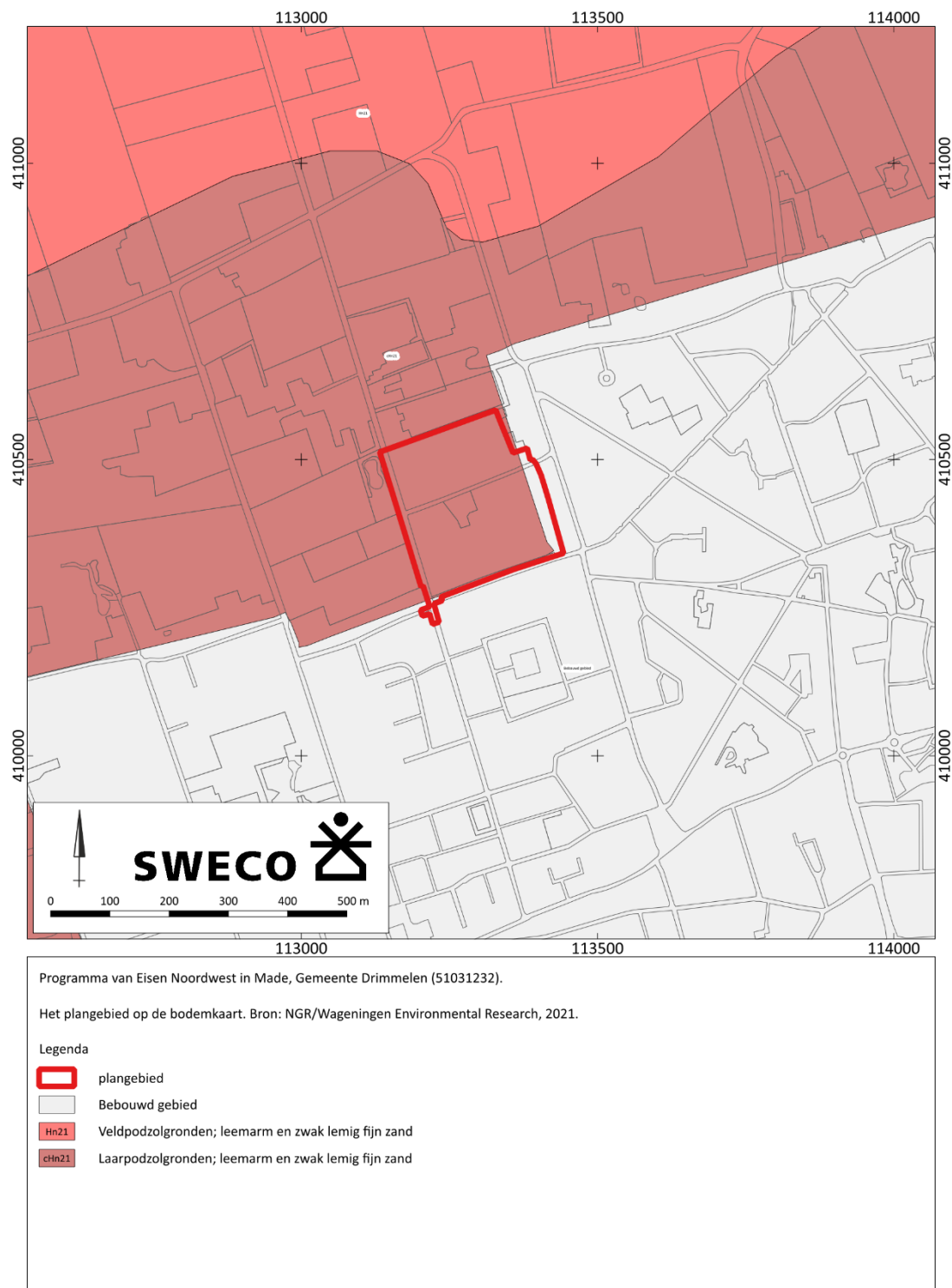
Figuur 6: Het plangebied op de bodemkaart van Nederland. 9
