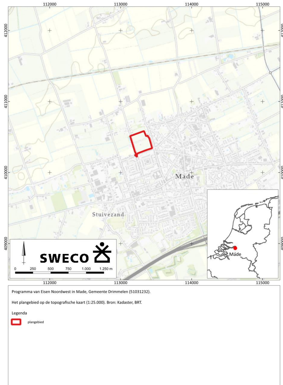
Figuur 1: Het plangebied op de topografische kaart (1:25.000).
