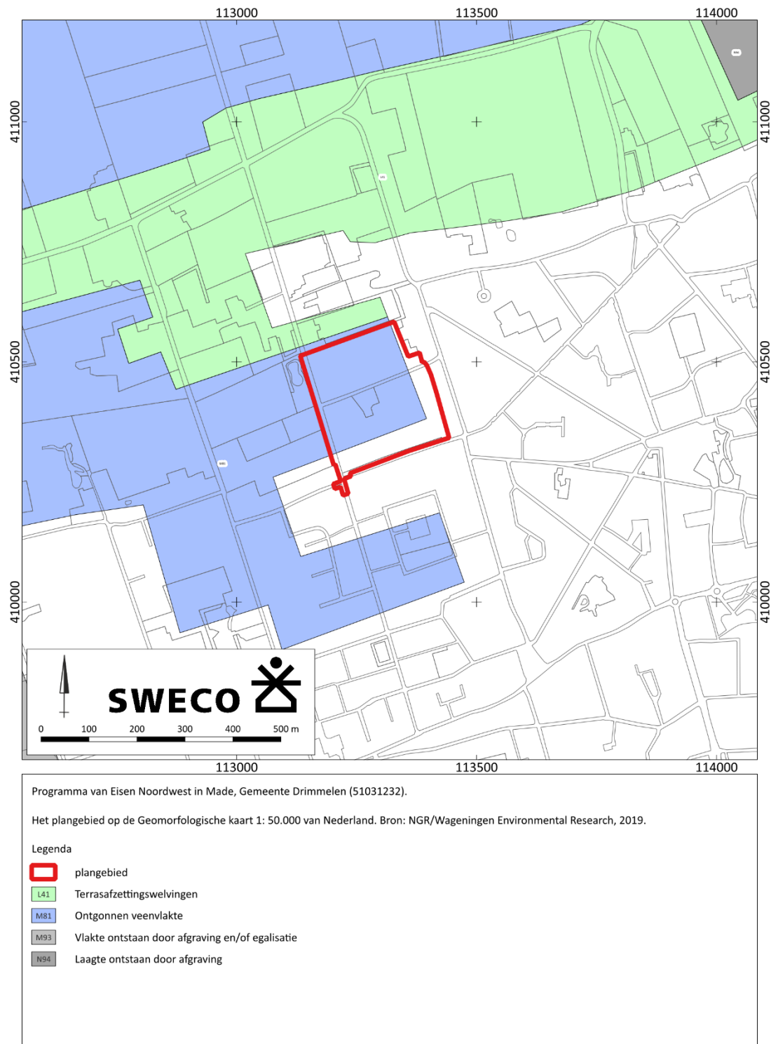
Figuur 5: Het plangebied op de Geomorfologische kaart van Nederland. 8
