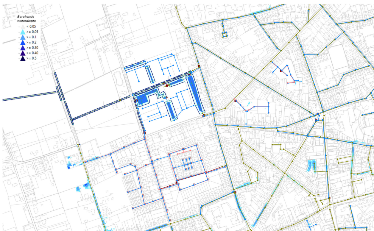
Figuur 4-3: Berekend water-op-sstraat Made Noordwest bij hydraulische ontwerpbui 09.
