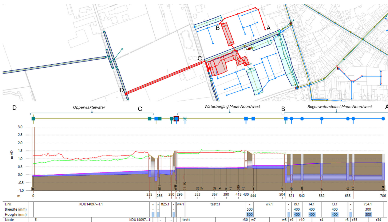
Figuur 4-5: Afvoercapaciteit regenwaterriolering Made Noordwest noordelijke route bij Bui 09.
