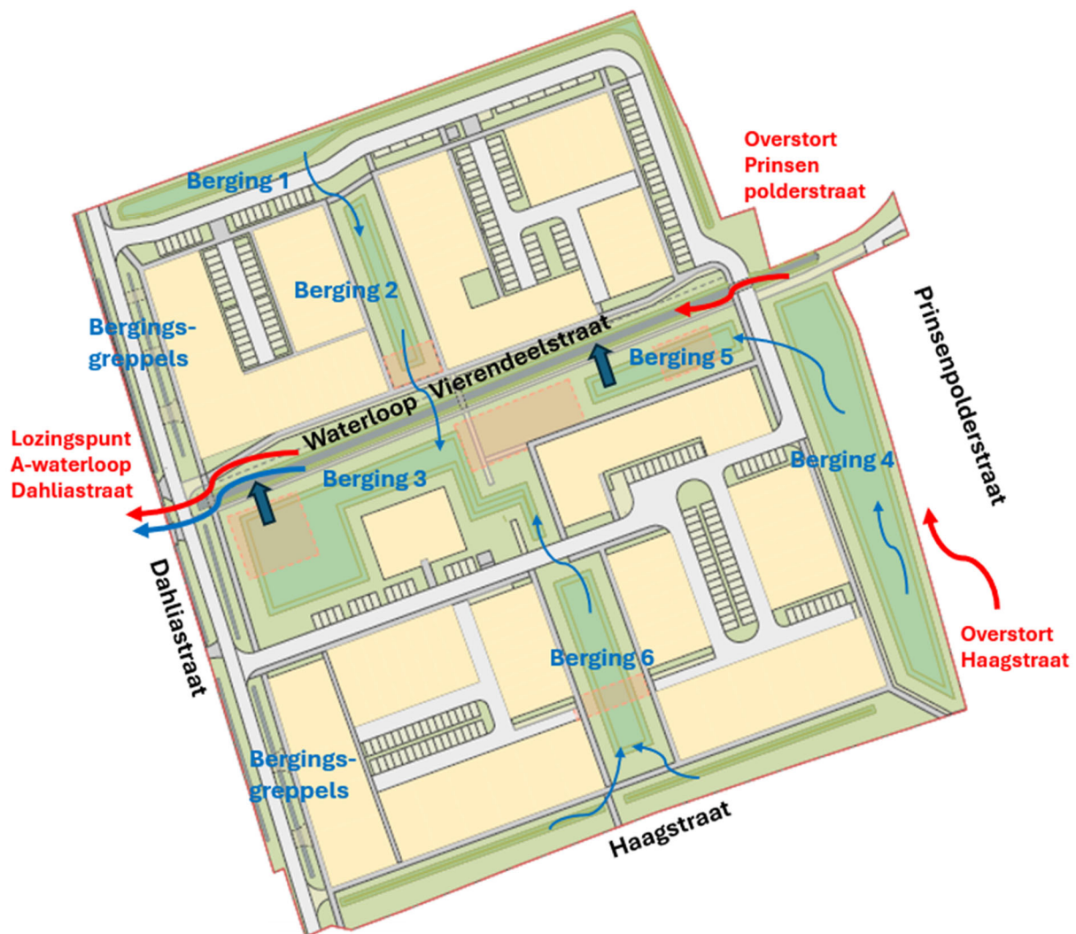
Figuur 1-2: Routekaart functioneel rioleringsontwerp Made Noordwest.
