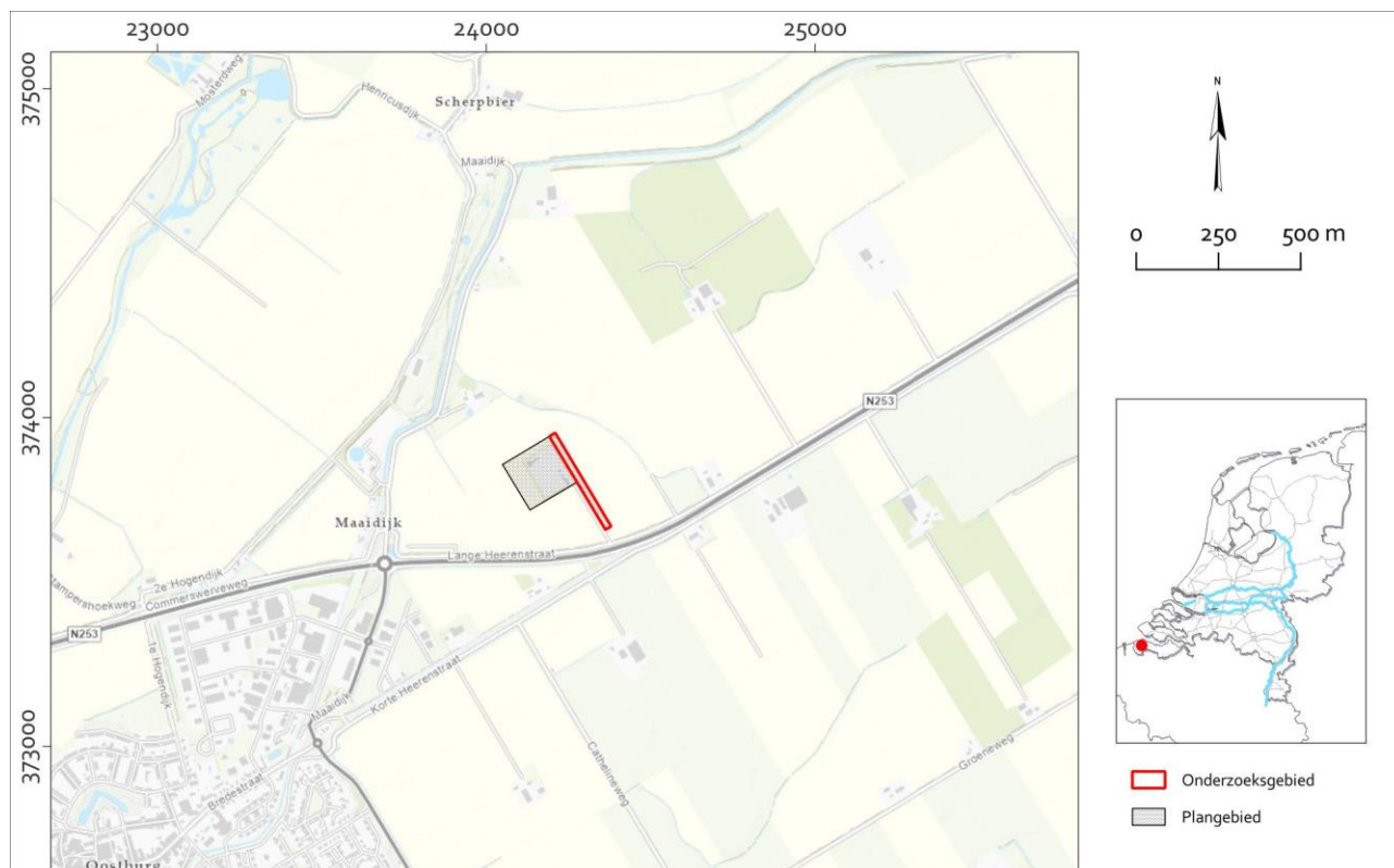
Figuur 1 Ligging van het plangebied in Nederland, schaal 1:25.000. Bron: ESRI Nederland, Community Map Contributors 2024.
