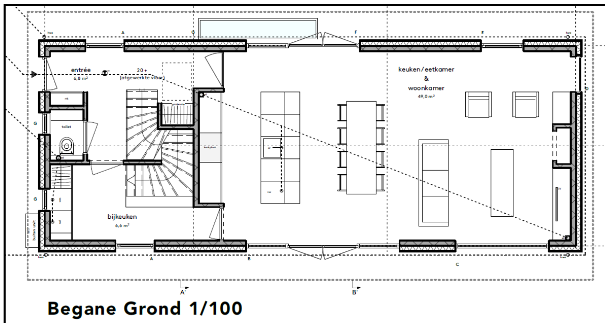
Figuur 4: Plattegrond begane grond nieuwe situatie
