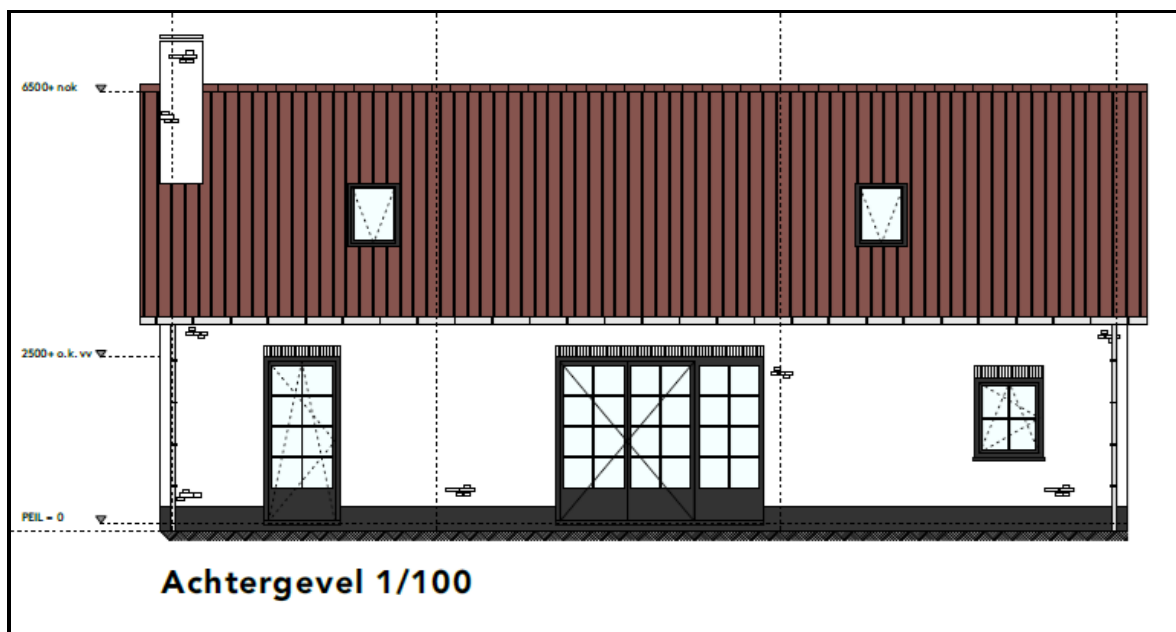
Figuur 3: Achtergevel nieuwe situatie
