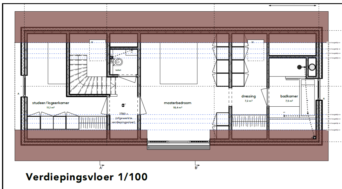
Figuur 5: Plattegrond 1 e verdieping nieuwe situatie
