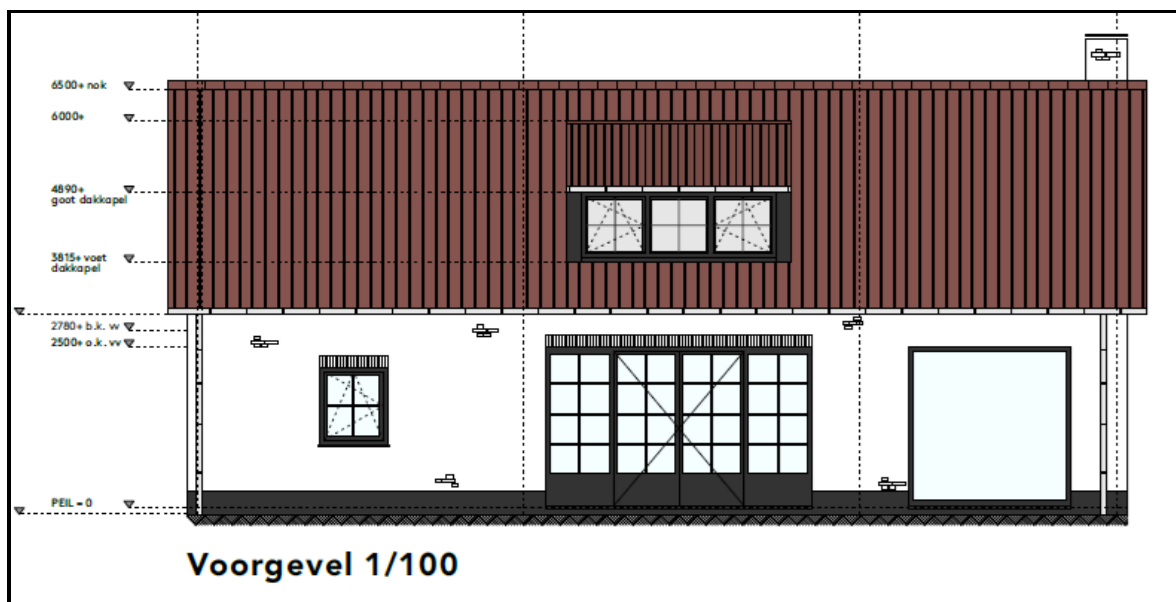
Figuur 2: Voorgevel nieuwe situatie
