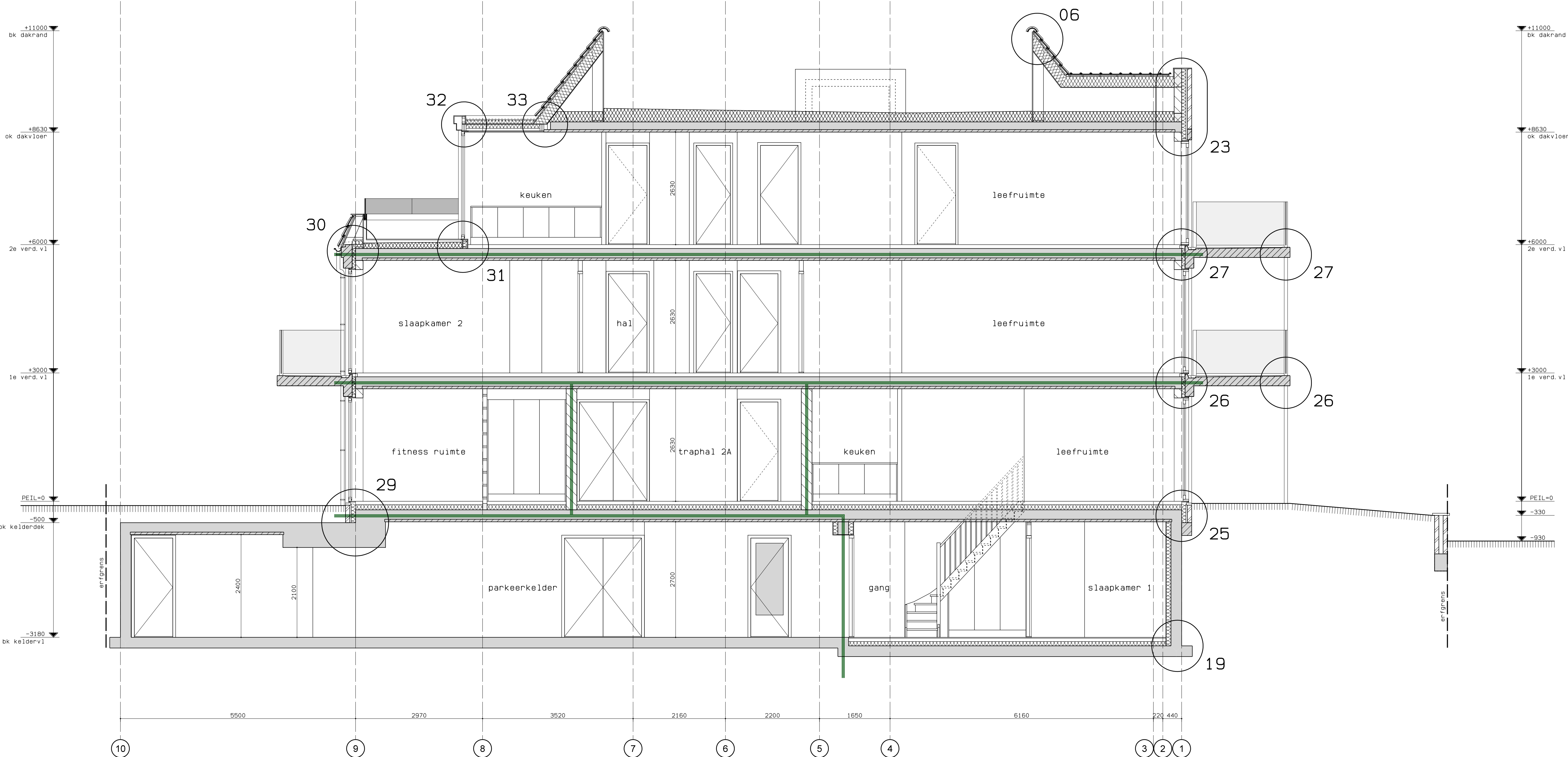
doorsnede D-D
