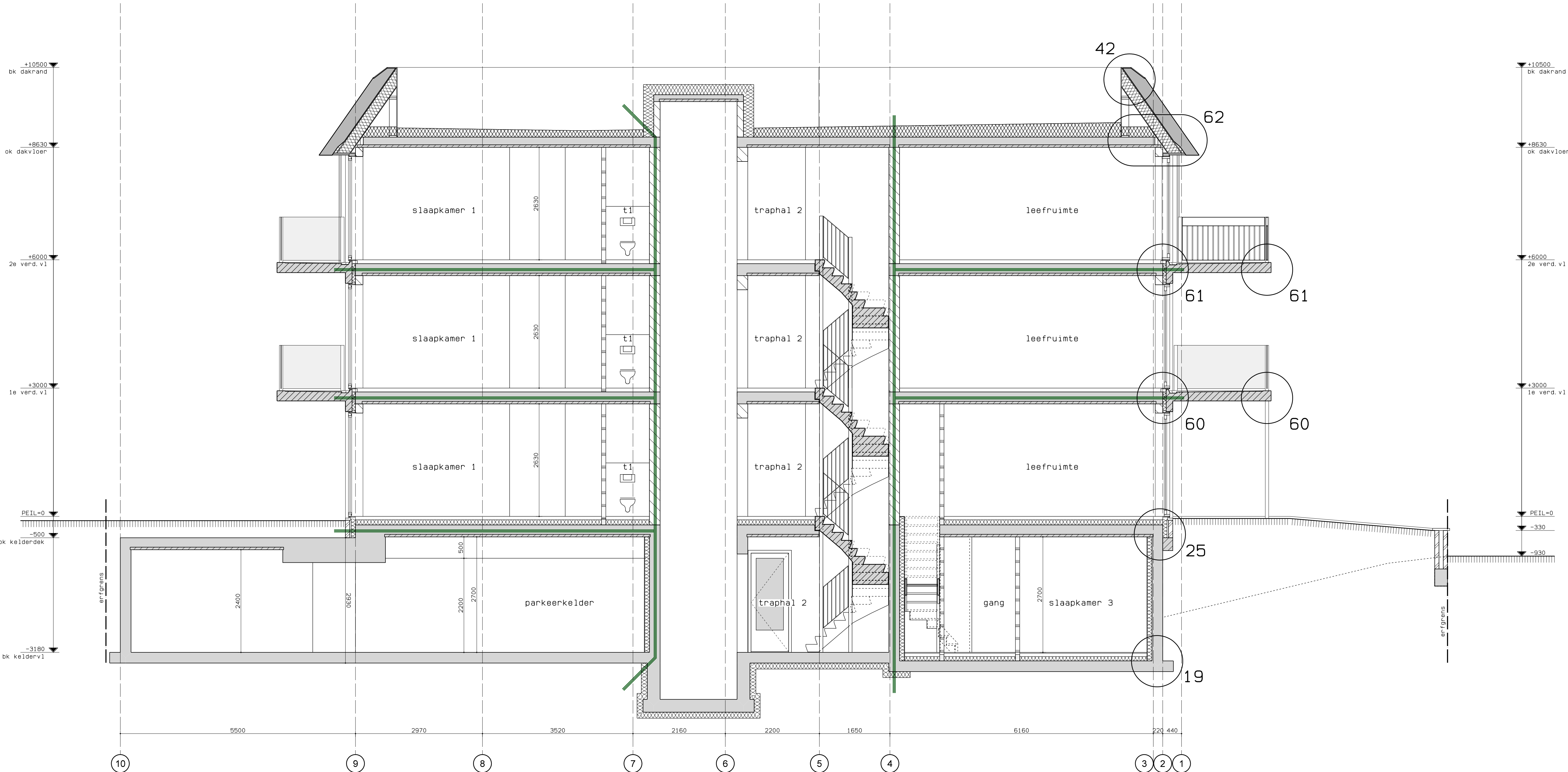
doorsnede A-A
