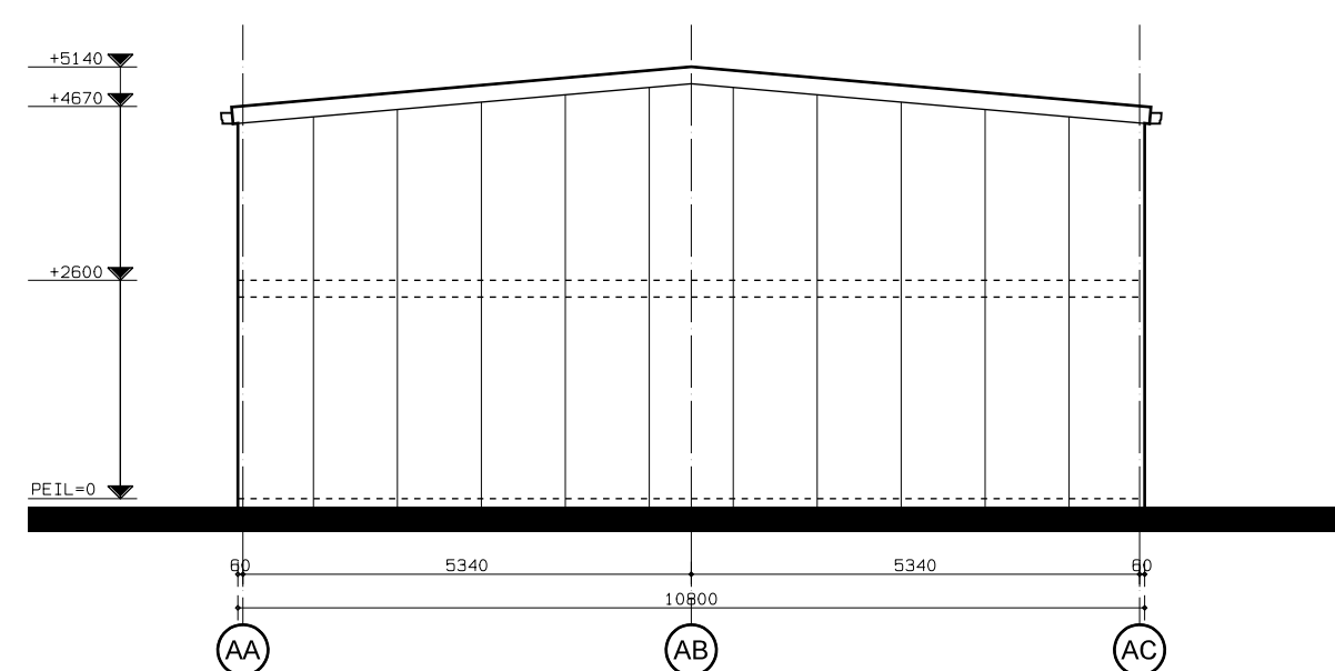
rechter zijgevel
