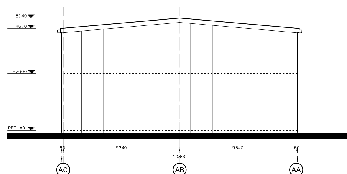
linker zijgevel
