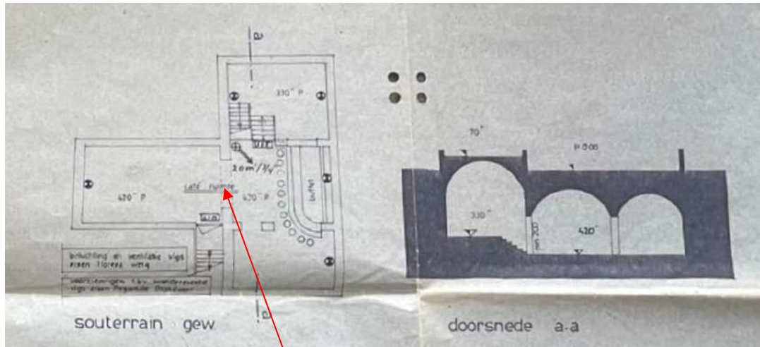
Afb. 48 Bouwtekening 1984
