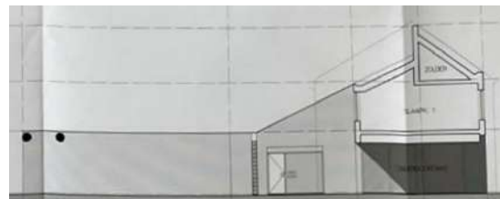
Afb. 65 Zijgevel aanzicht nieuw 2011
