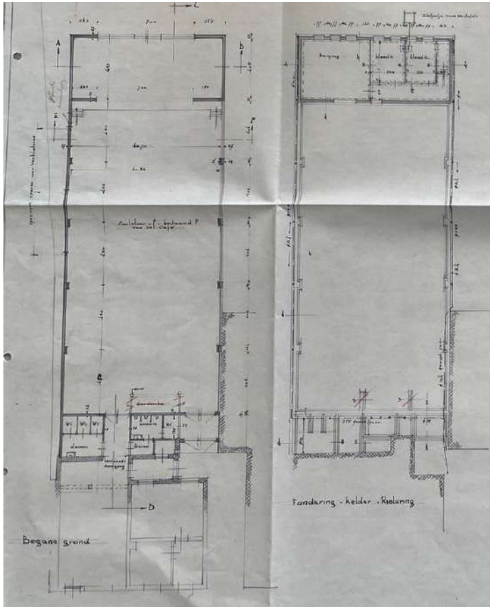
Afb. 19 bouwtekening 1958
