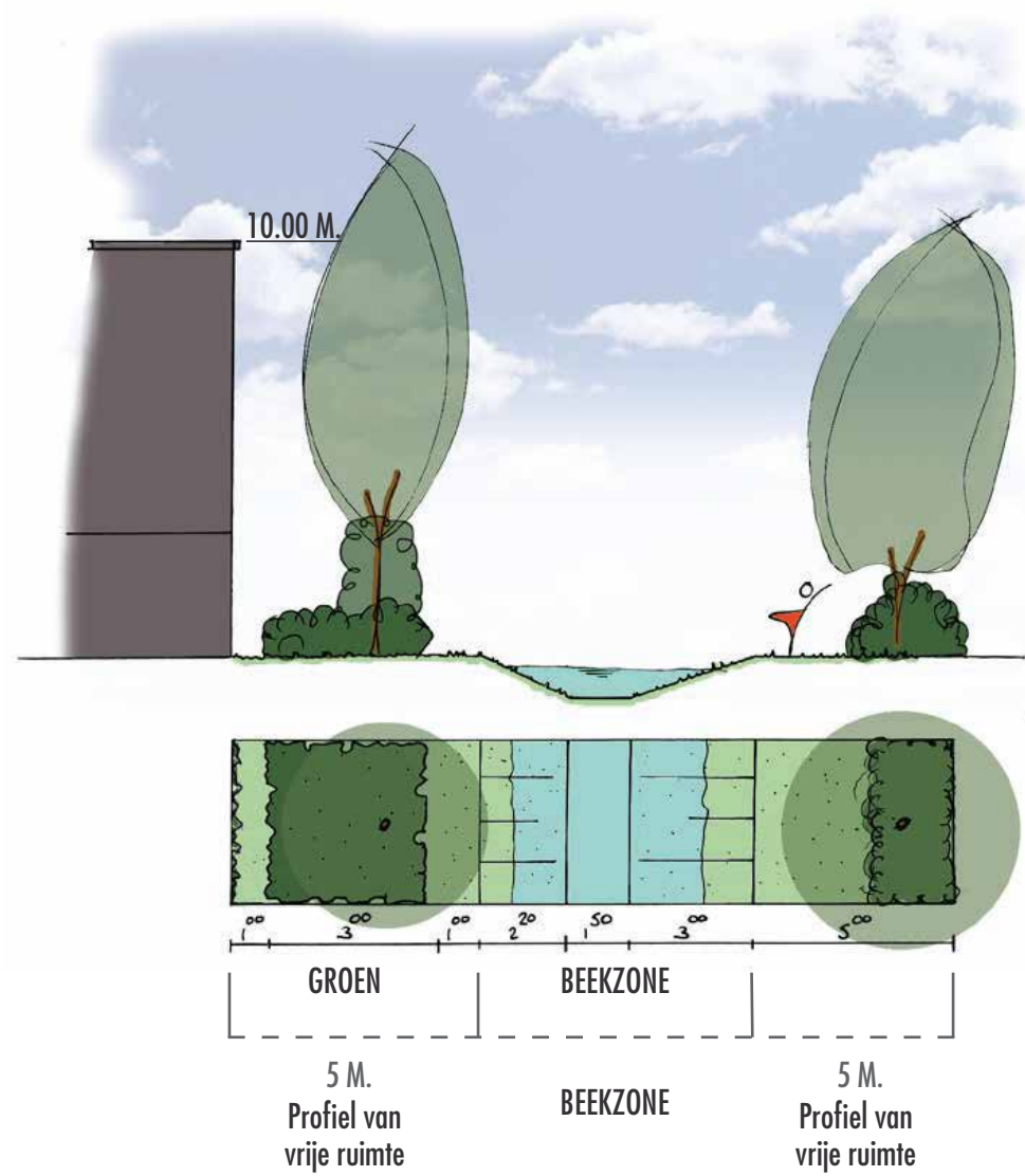
PROFIEL 1: AANSLUITING BEDRIJFSGEBOUW MET BEEKZONE EXCLUSIEF MUUR
