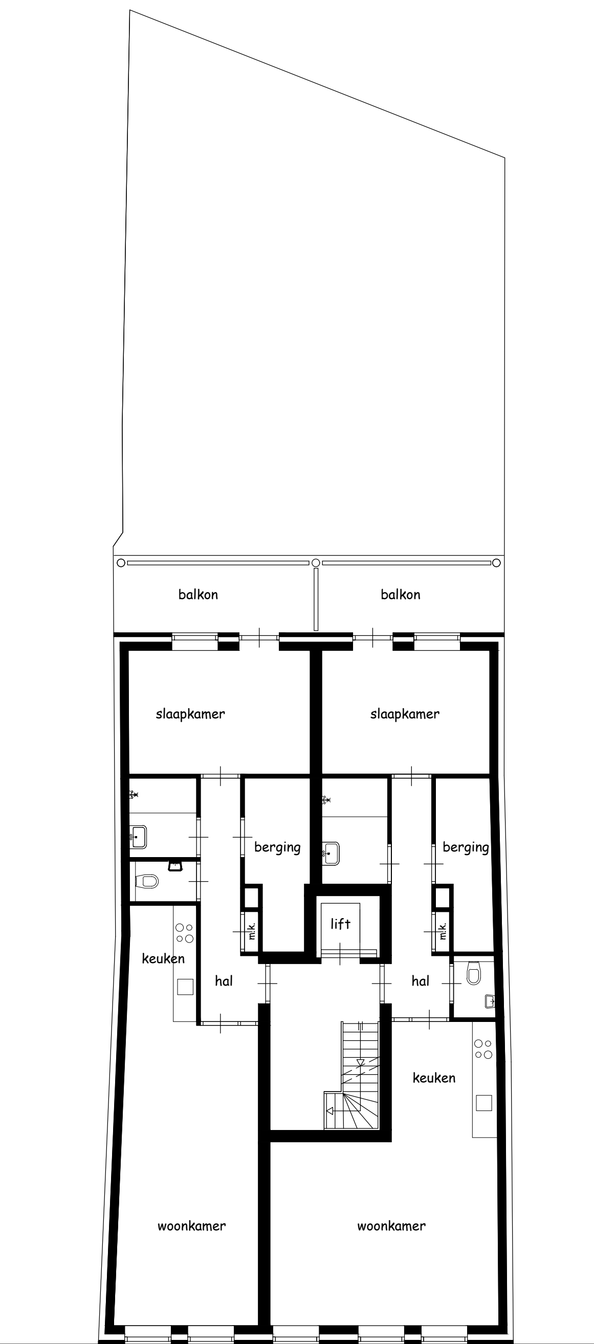
1e verdieping
