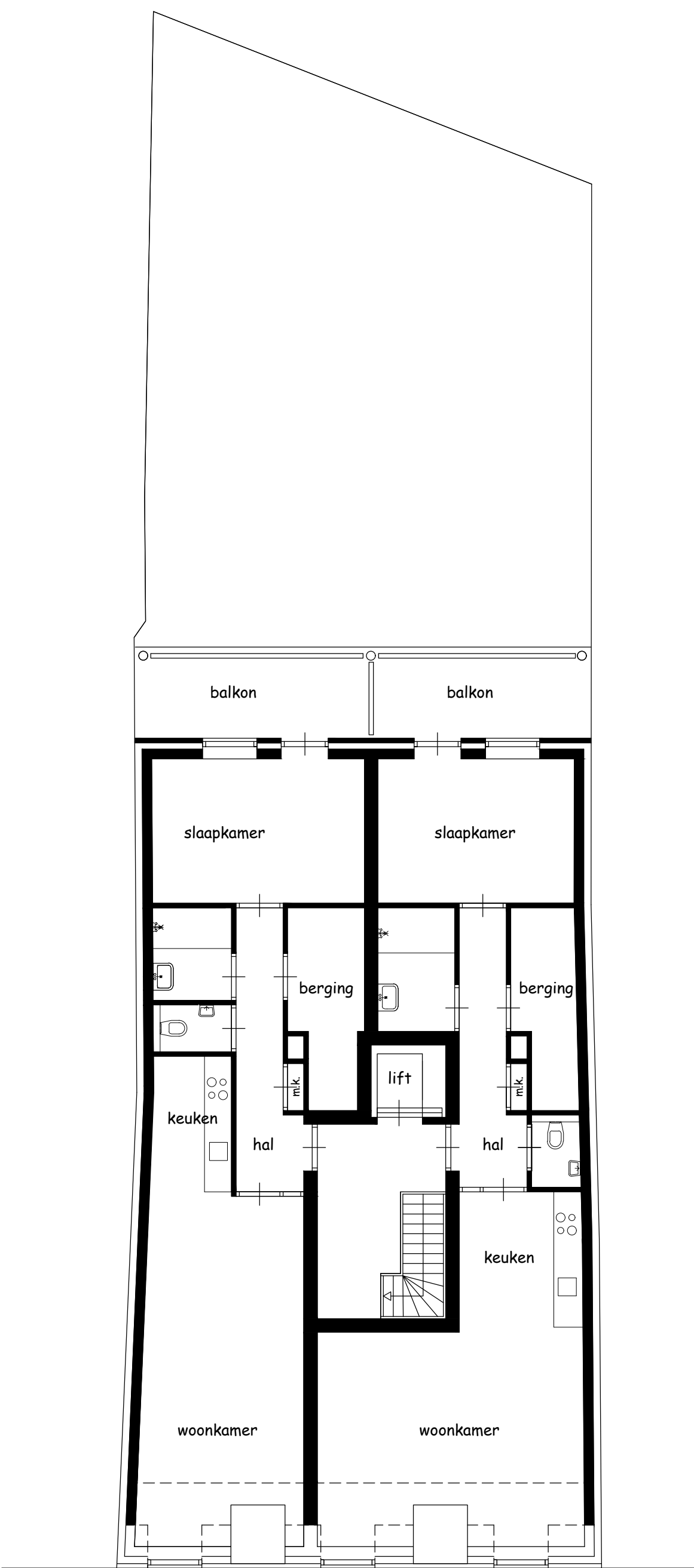
2e verdieping
