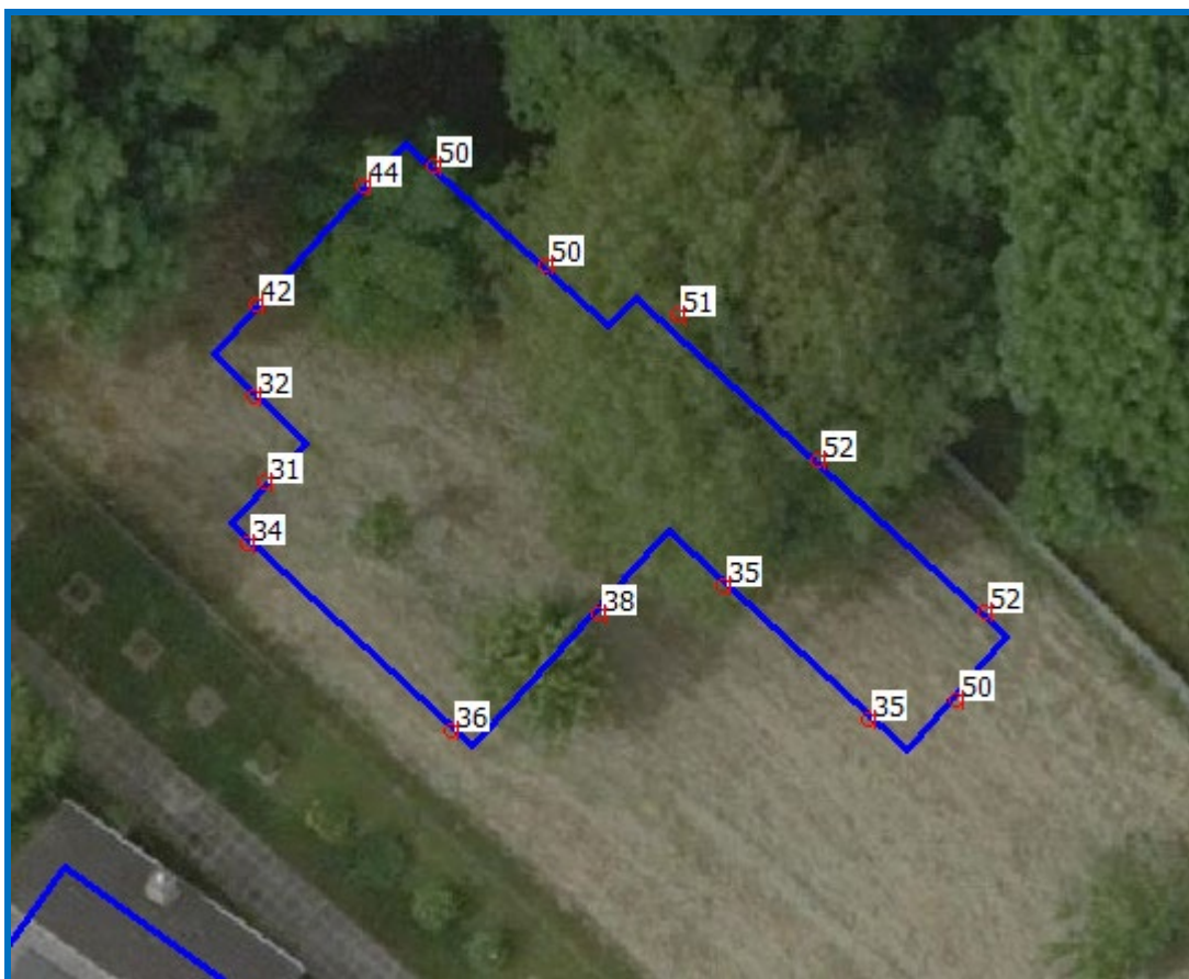
Figuur H: langtijdgemiddelde beoordelingsniveaus in dB(A) in de avondperiode incidentele situatie
