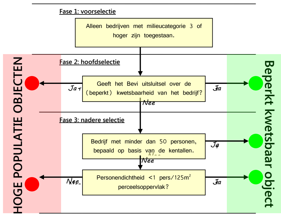
Figuur B4.3: stroomschema kwetsbaarheidbepaling.
