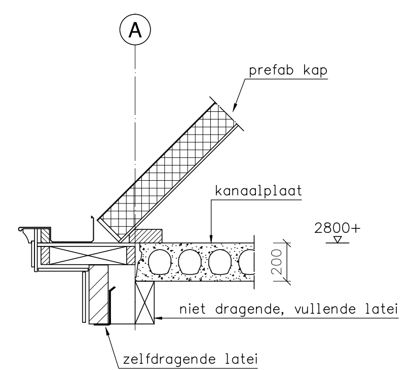
Doorsnede C
