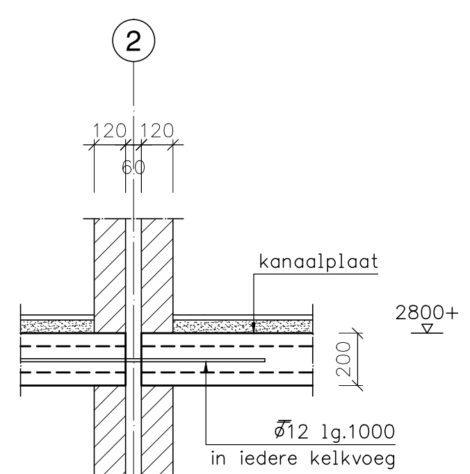
Doorsnede B
