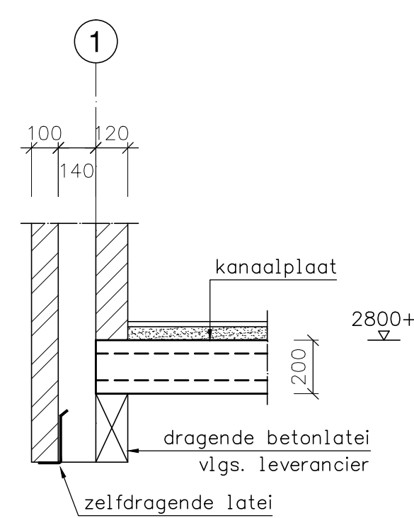
Doorsnede A
