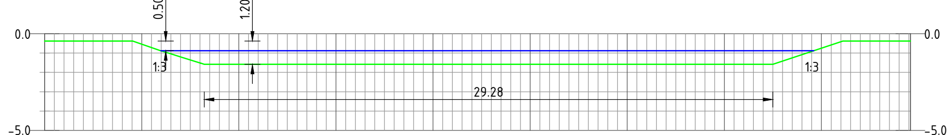
Profiel B-B
