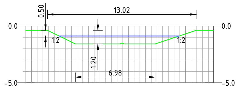
Profiel A-A
