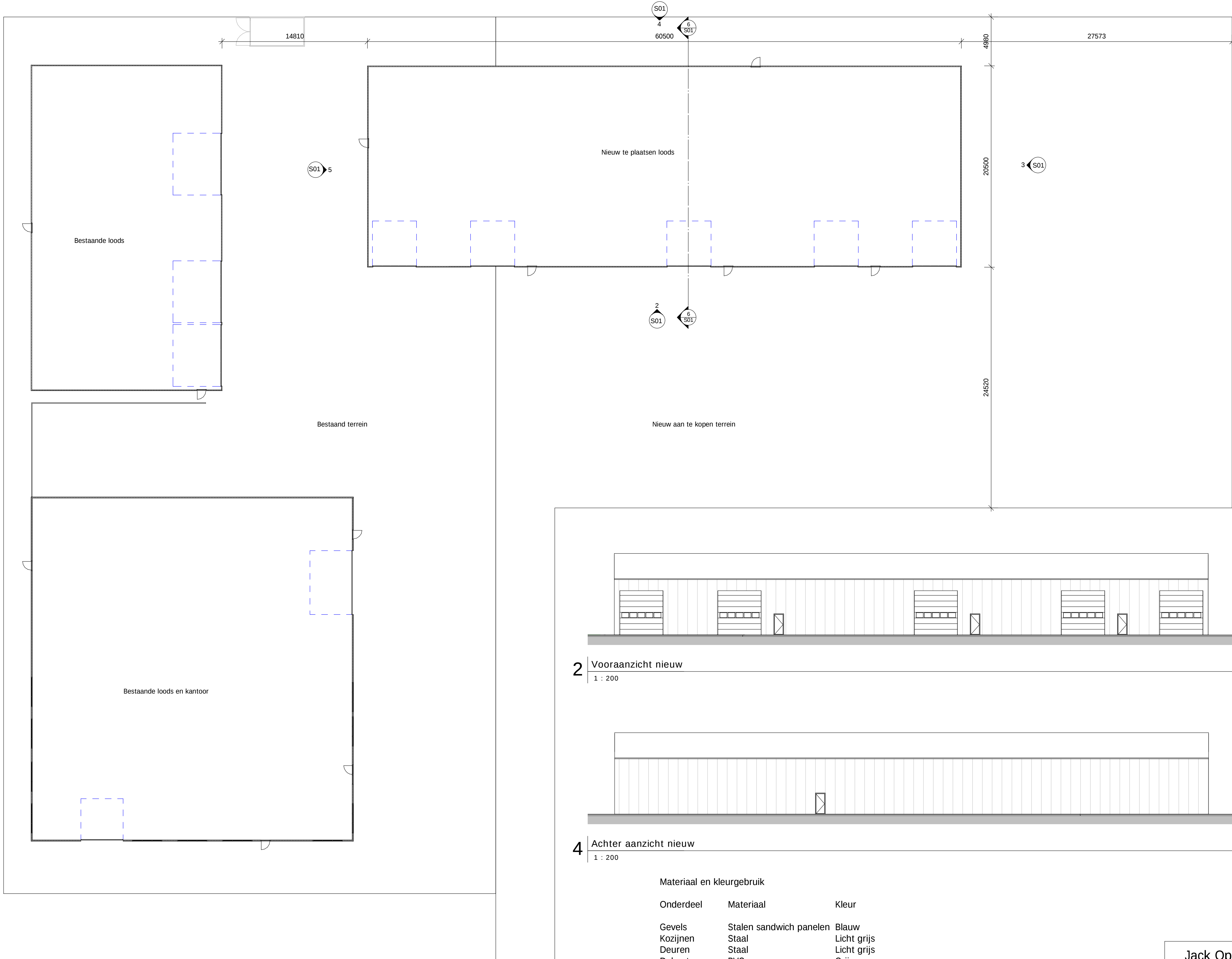
1 Begane grond nieuw 1 : 200
