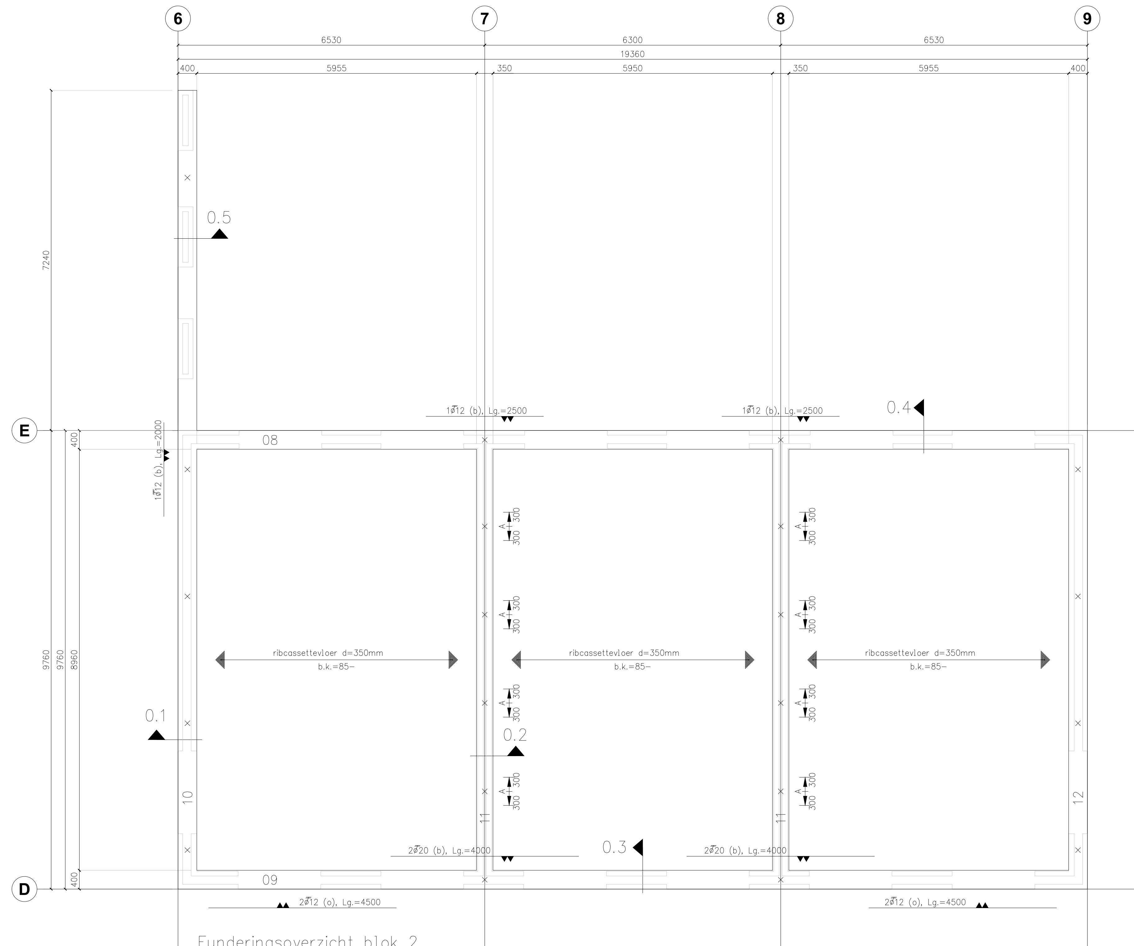
Funderingsoverzicht blok 2
