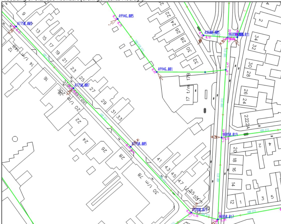
Afbeelding 3. Uitsnede rioolkaart (bron: gemeente Moerdijk).
