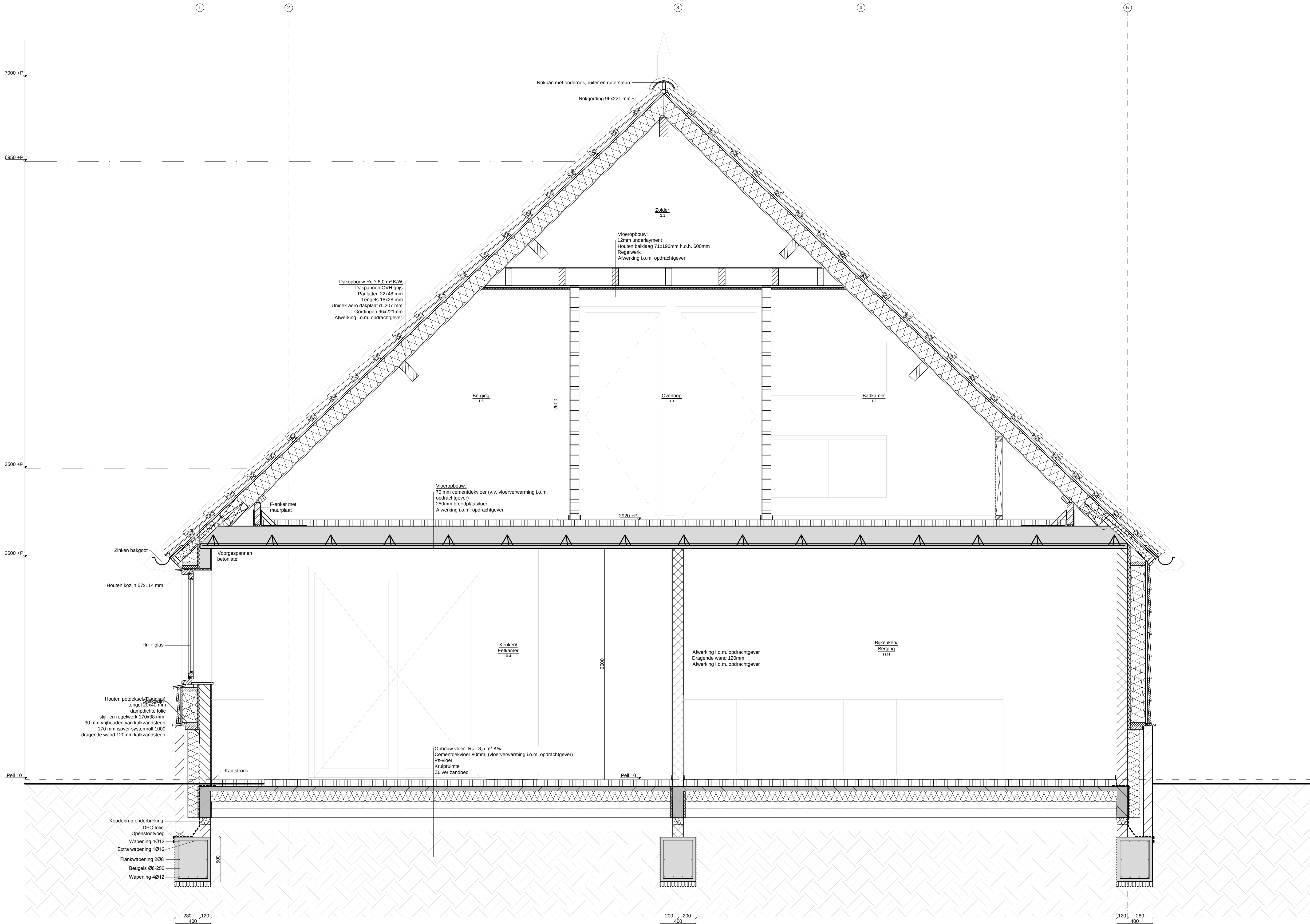
Doorsnede B-B
