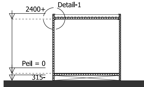
- doorsnede B-B -
