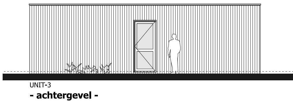
- achtergevel -
