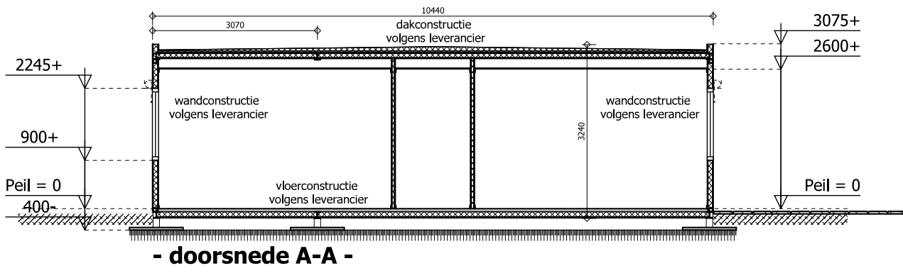
- doorsnede A-A -
