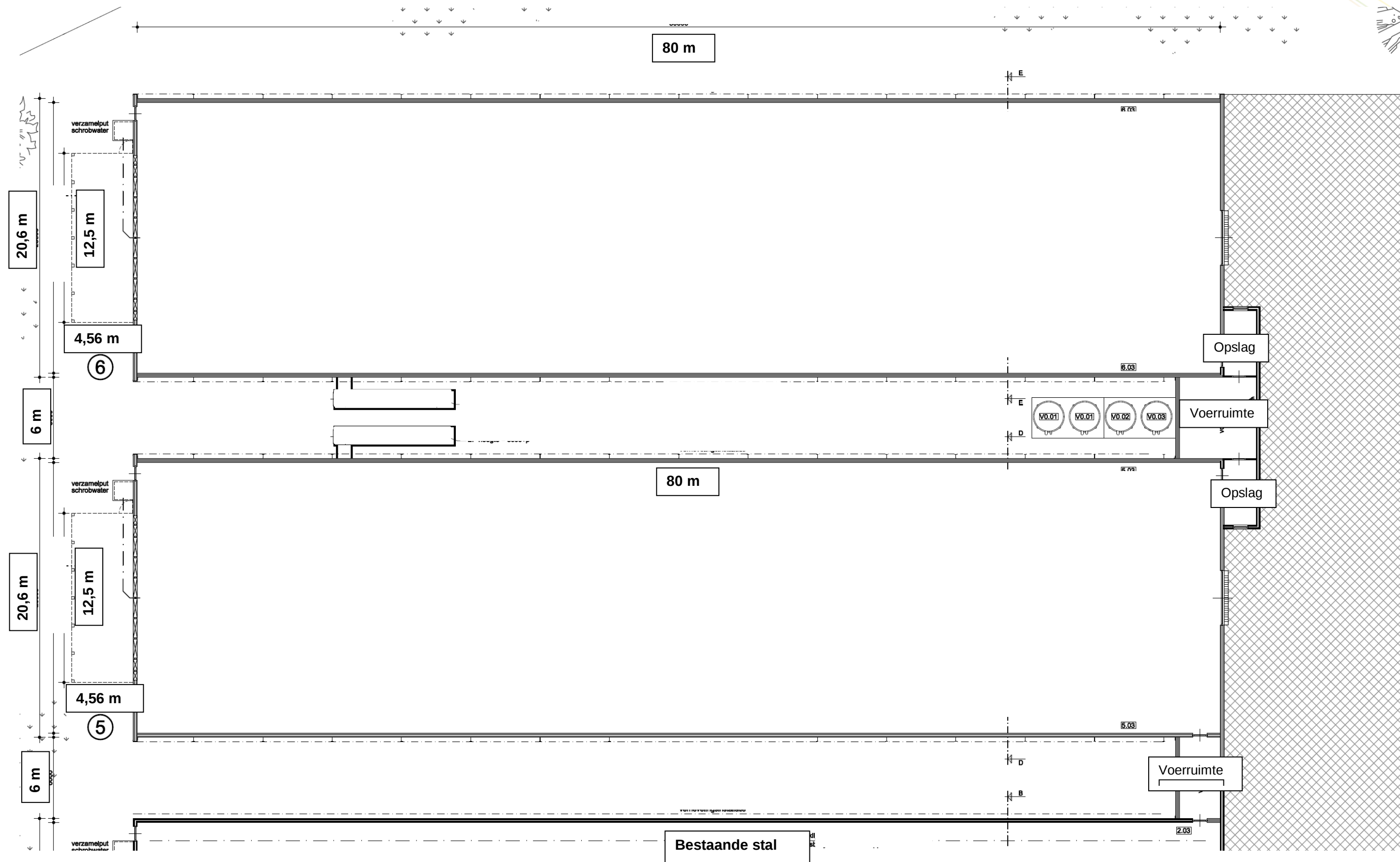
Bijlage 8. Weergave gewenste situatie inclusief maatvoeringen Koekoekendijk 10 te Moerdijk
