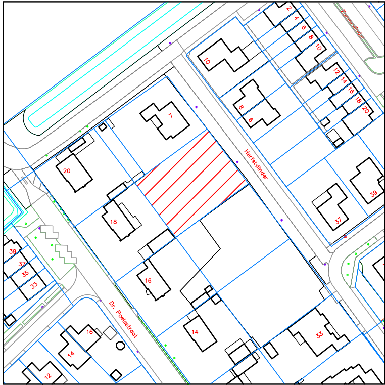
overzichtskaart schaal: 1 : 4000
