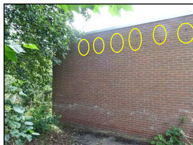
Figuur 13. Open stootvoegen aanwezig in de buitenmuur.
