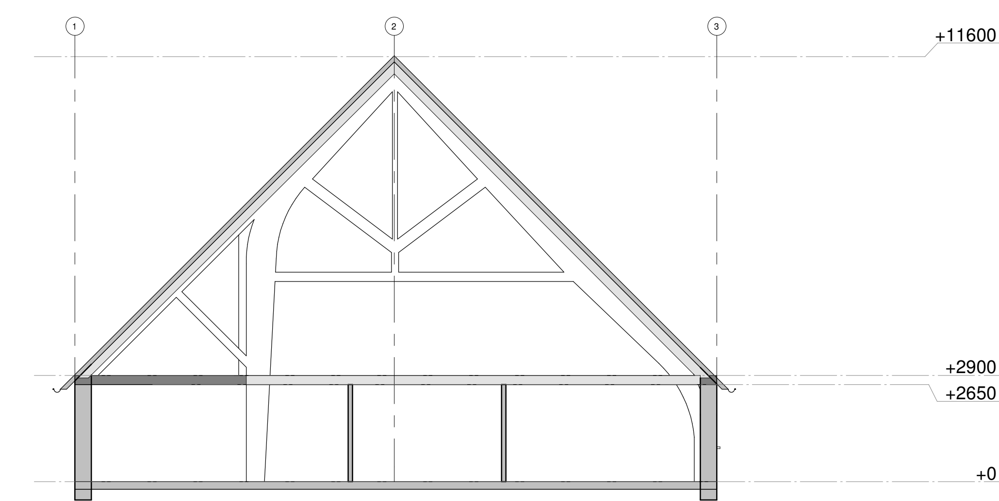
doorsnede
