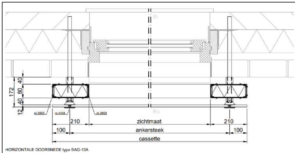
Figuur 2: voorbeelddetailering SilentAir-gevelschermb (bron: Metaglas)
