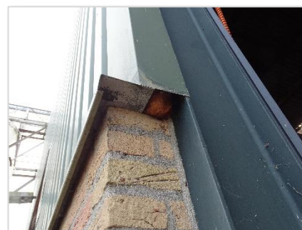
Foto 16: Pand 2 – gevel (randen dicht).
