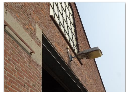
Foto 39: Pand 5 – kieren en openingen bij dakrand zuidzijde.
