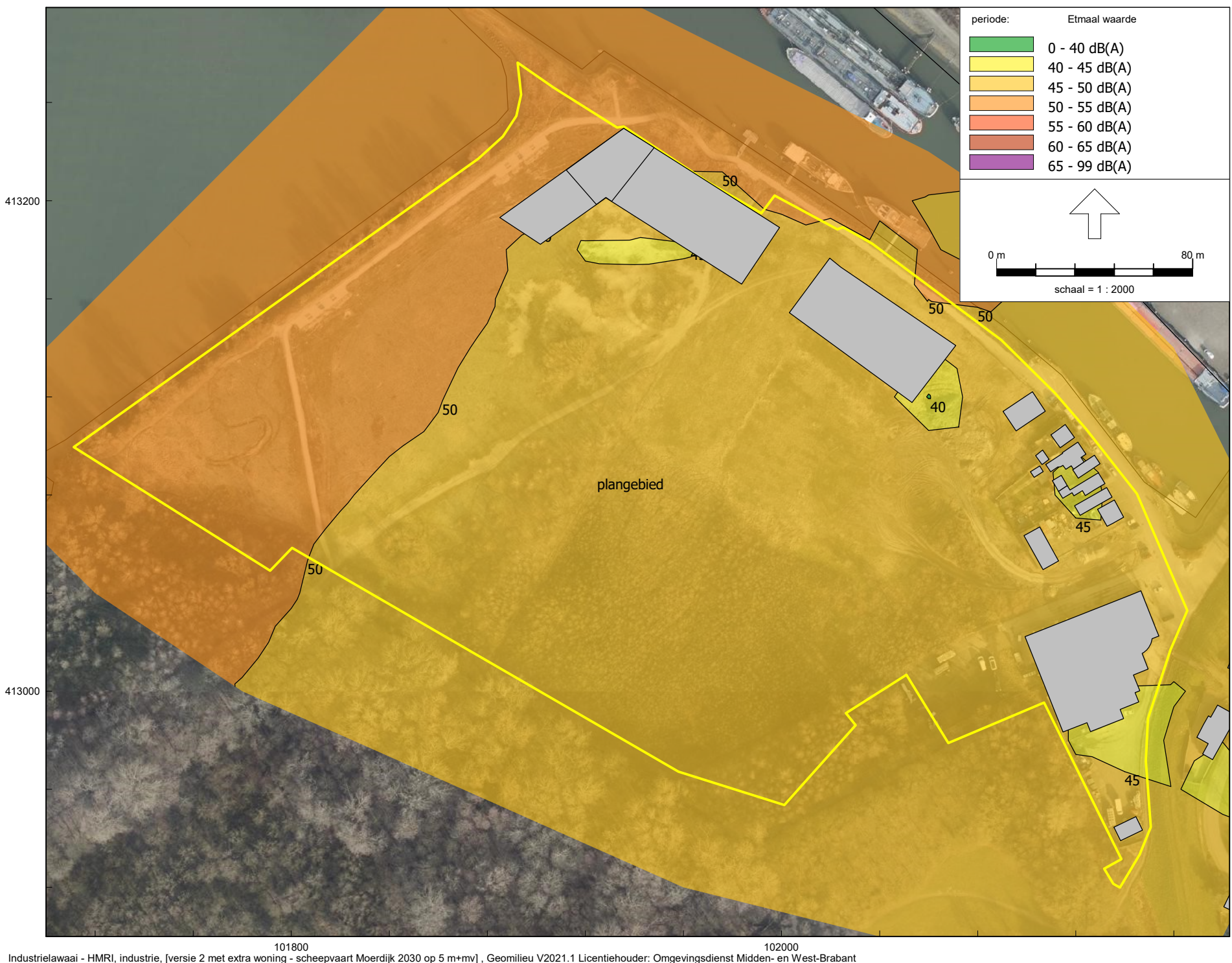
Figur 18 Rekenresultaten scheepvaart op 5 m+mv Omgevingsdienst Midden- en West-Brabant
