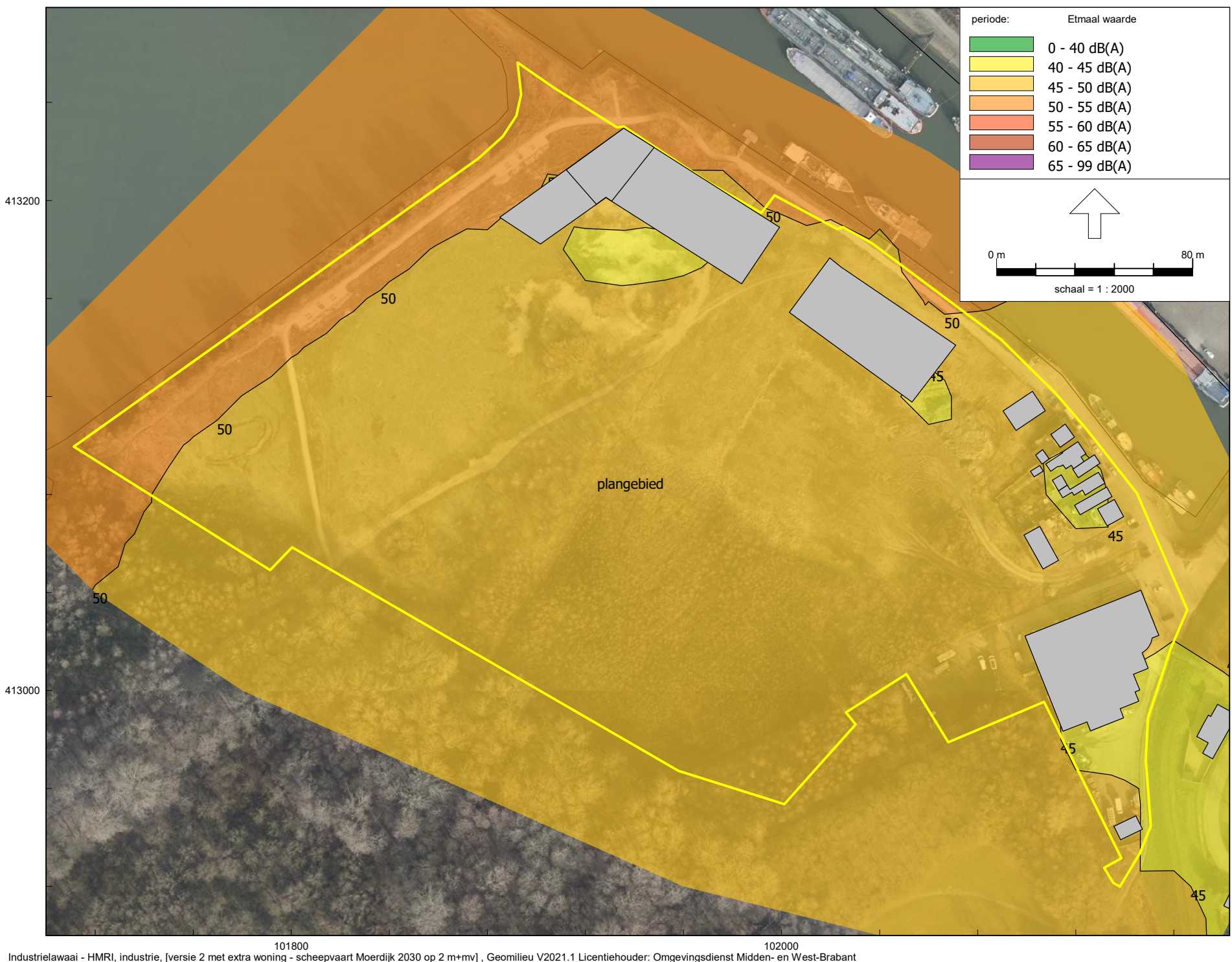
Figur 18 Rekenresultaten scheepvaart op 2 m+mv
