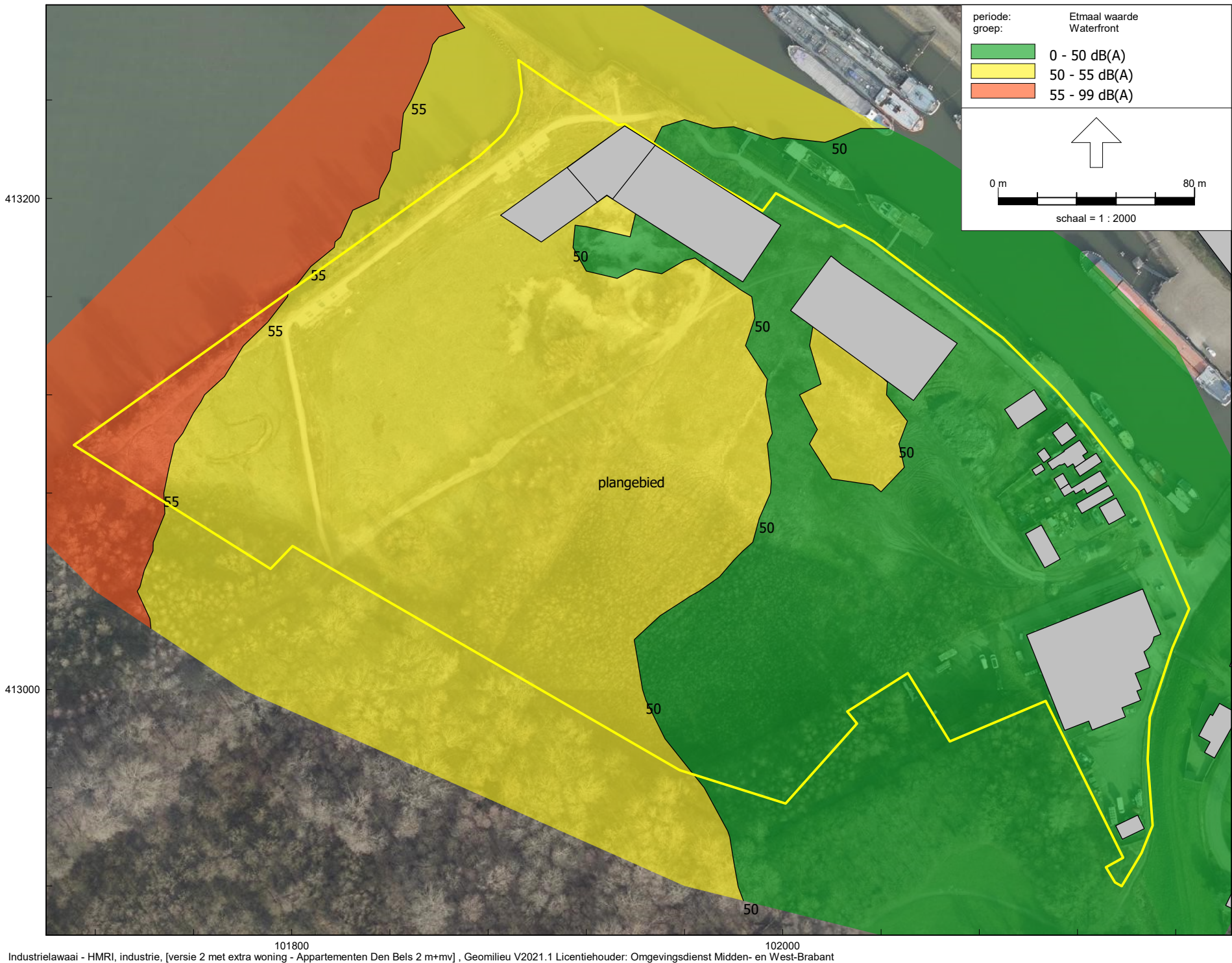
Figuur 19 Rekenresultaten industrielaawaai op 2 m+mv Omgevingsdienst Midden- en West-Brabant
