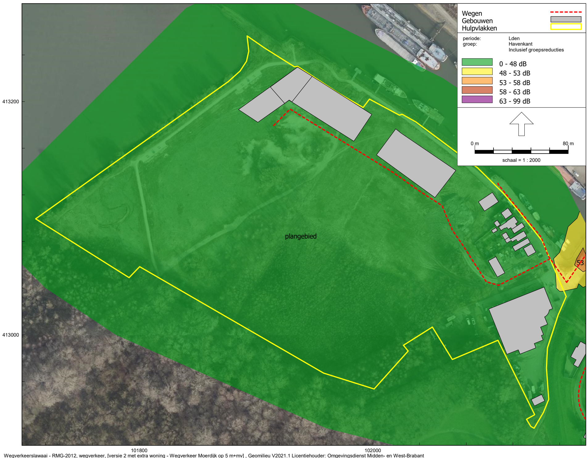
Figur 14 Rekenresultaten Havenkant op 5 m+mv Omgevingsdienst Midden- en West-Brabant
