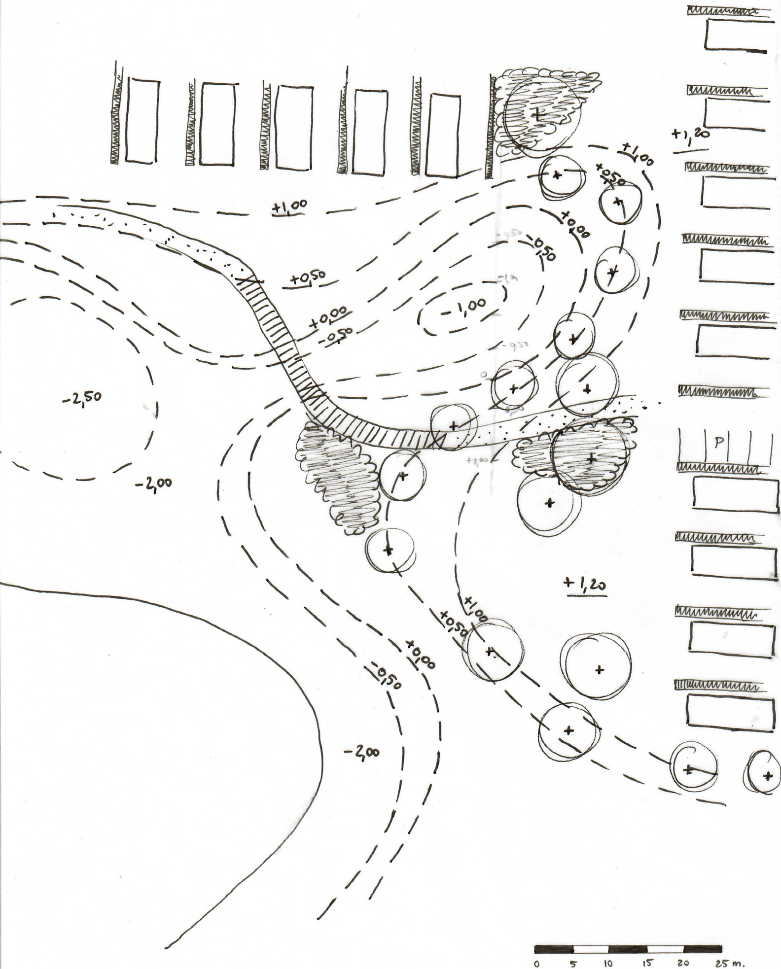
aanpassing moeraszone 1:500
