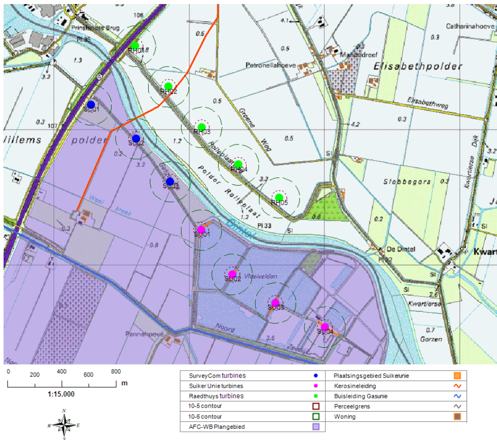
Figuur 1 Plattegrond met indicatie van de windturbines van de drie initiatieven van Windpark Dintel
